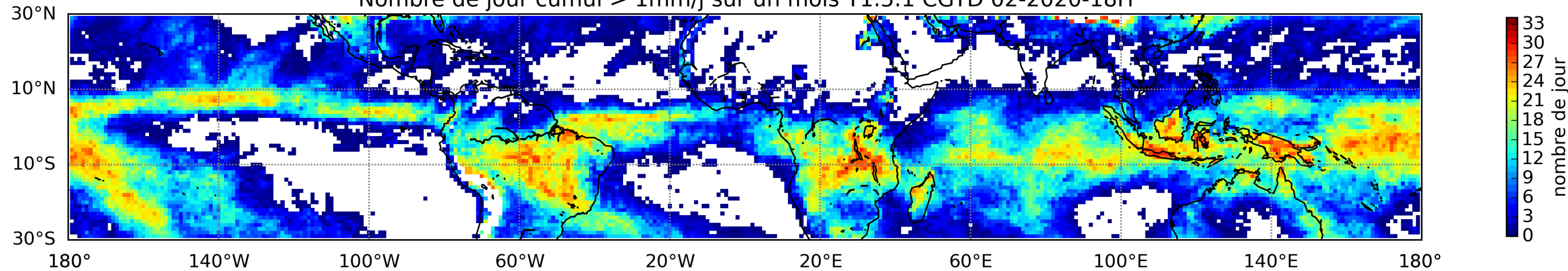
Nombre de jour cumul > 1mm/j sur un mois T1.5.1 CGTD 02-2020-18H
