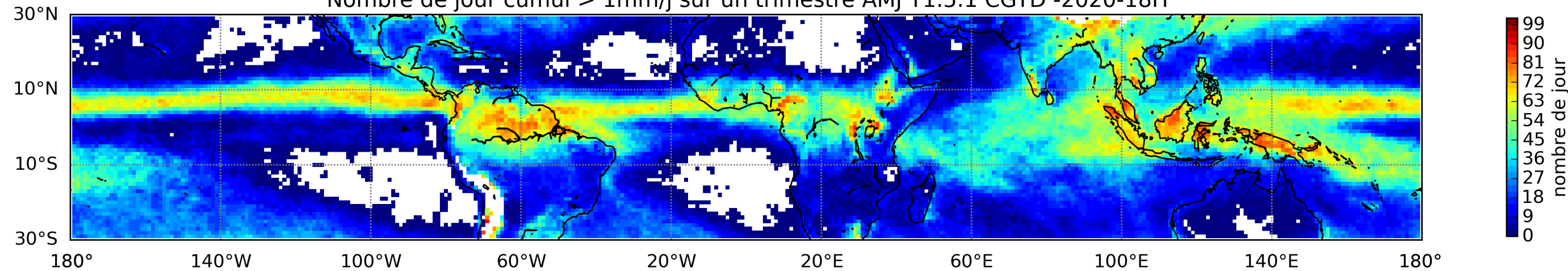
Nombre de jour cumul > 1mm/j sur un trimestre AMJ T1.5.1 CGTD -2020-18H
