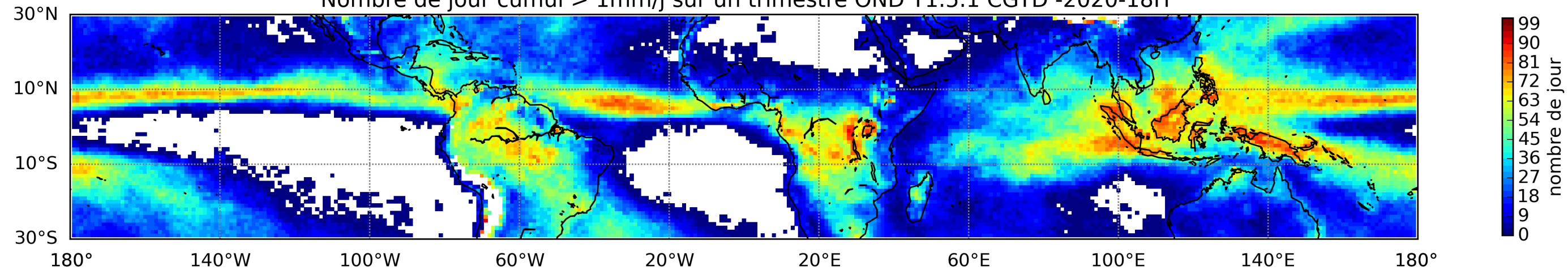
Nombre de jour cumul > 1mm/j sur un trimestre OND T1.5.1 CGTD -2020-18H
