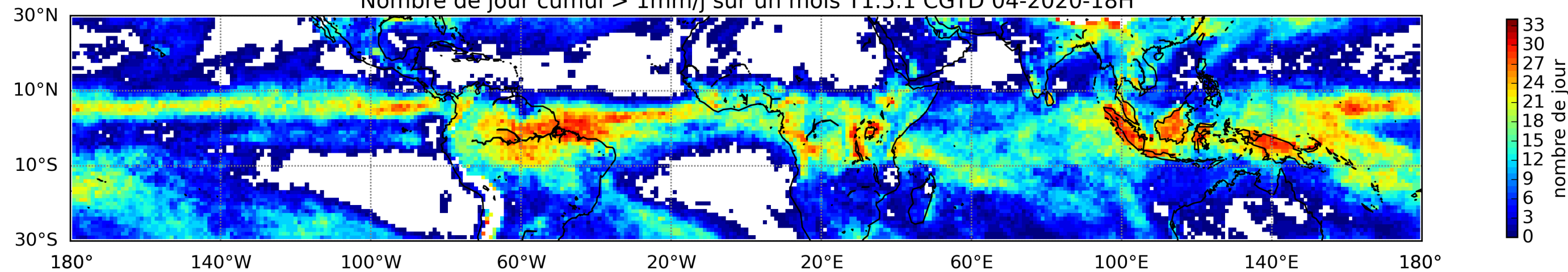
Nombre de jour cumul > 1mm/j sur un mois T1.5.1 CGTD 04-2020-18H
