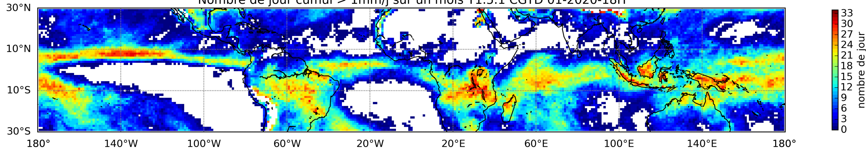
Nombre de jour cumul > 1mm/j sur un mois T1.5.1 CGTD 01-2020-18H
