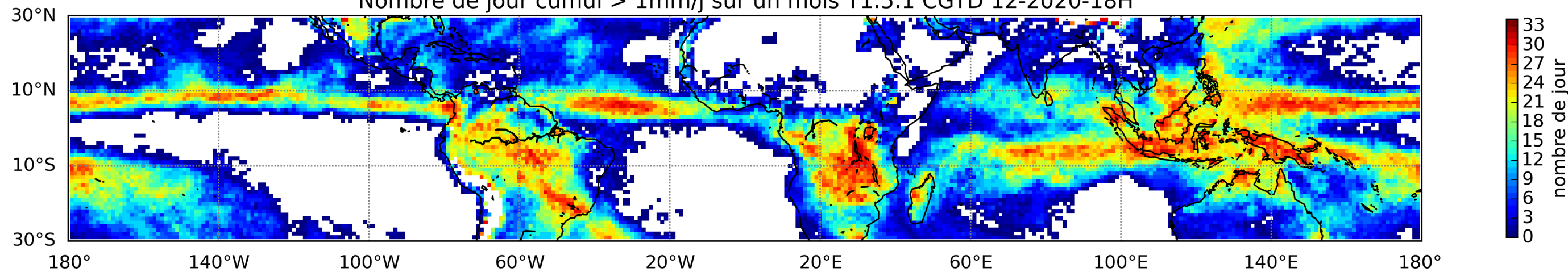
Nombre de jour cumul > 1mm/j sur un mois T1.5.1 CGTD 12-2020-18H
