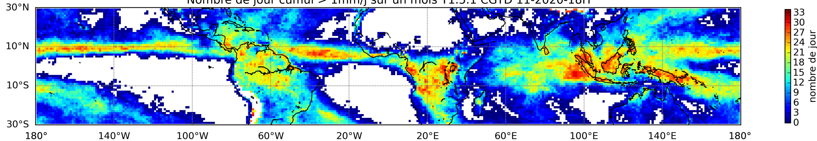
Nombre de jour cumul > 1mm/j sur un mois T1.5.1 CGTD 11-2020-18H
