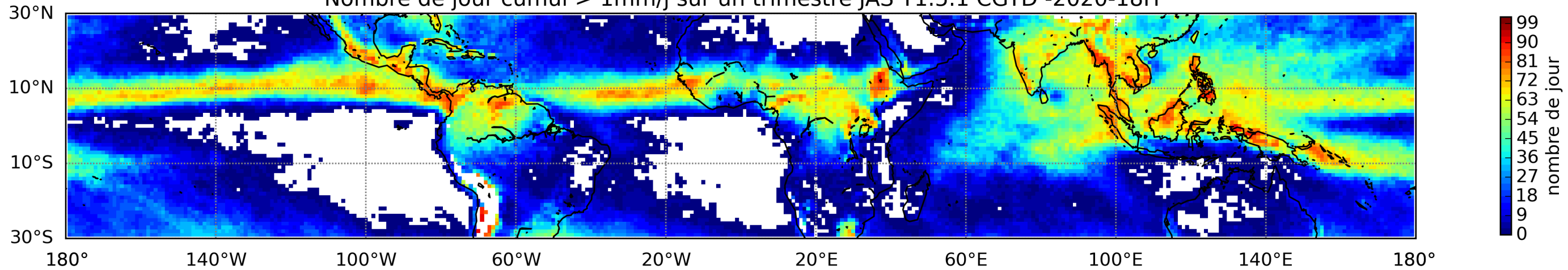
Nombre de jour cumul > 1mm/j sur un trimestre JAS T1.5.1 CGTD -2020-18H
