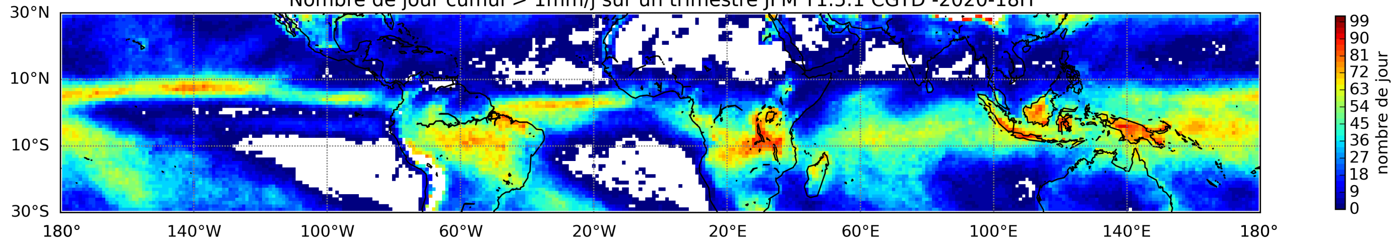
Nombre de jour cumul > 1mm/j sur un trimestre JFM T1.5.1 CGTD -2020-18H
