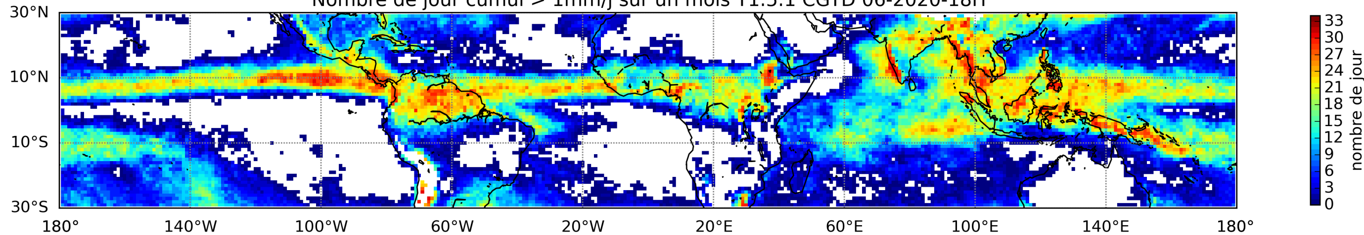
Nombre de jour cumul > 1mm/j sur un mois T1.5.1 CGTD 06-2020-18H
