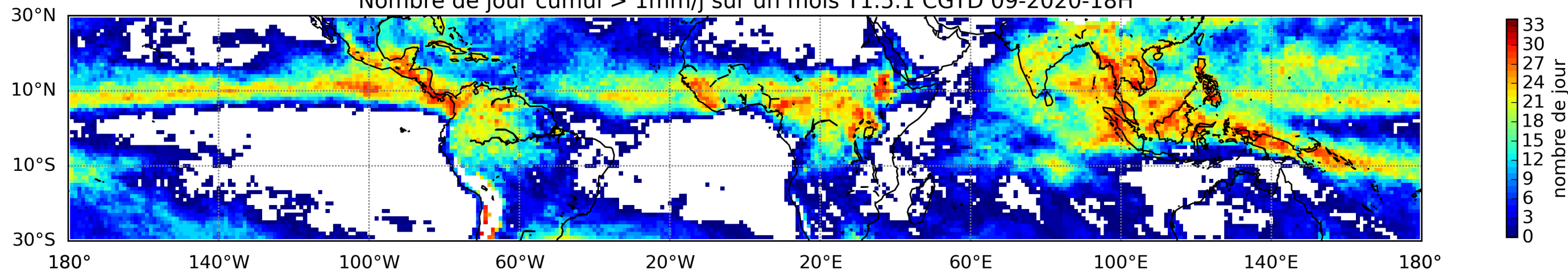
Nombre de jour cumul > 1mm/j sur un mois T1.5.1 CGTD 09-2020-18H
