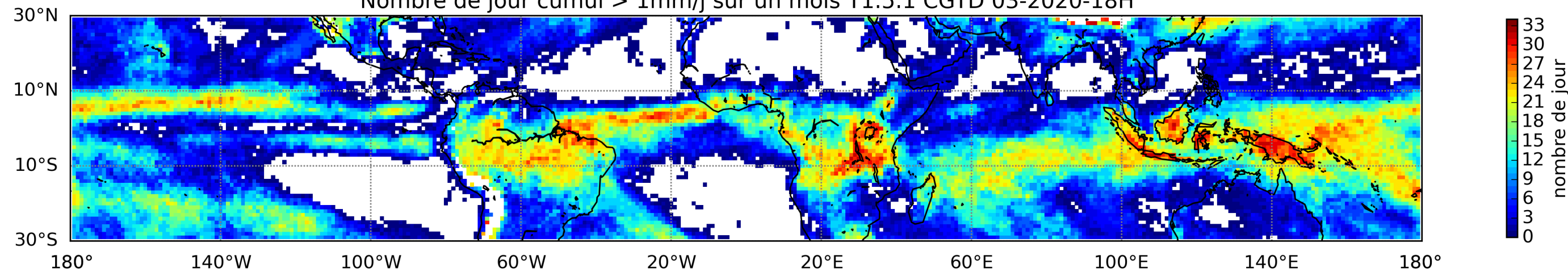
Nombre de jour cumul > 1mm/j sur un mois T1.5.1 CGTD 03-2020-18H
