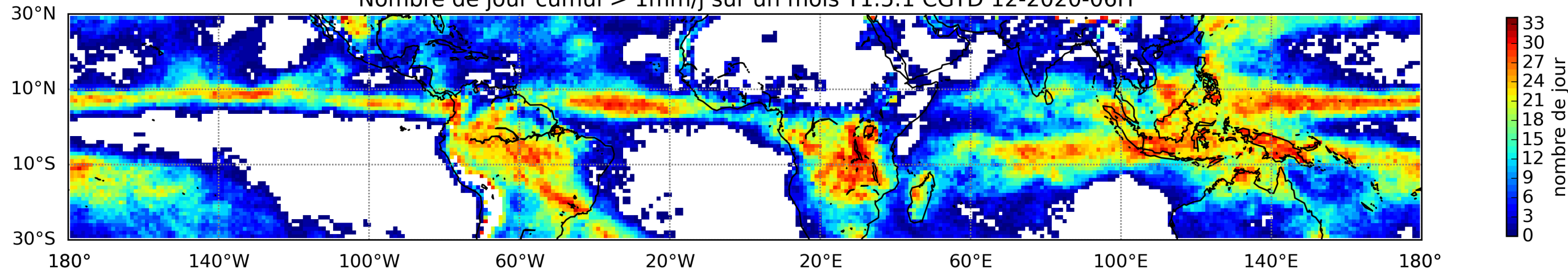
Nombre de jour cumul > 1mm/j sur un mois T1.5.1 CGTD 12-2020-06H
