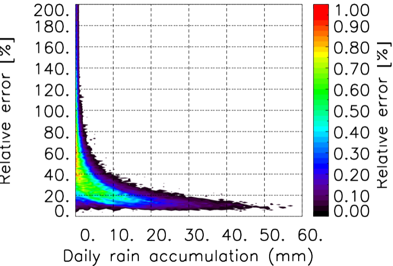
TERRE : 12 2020 00H
