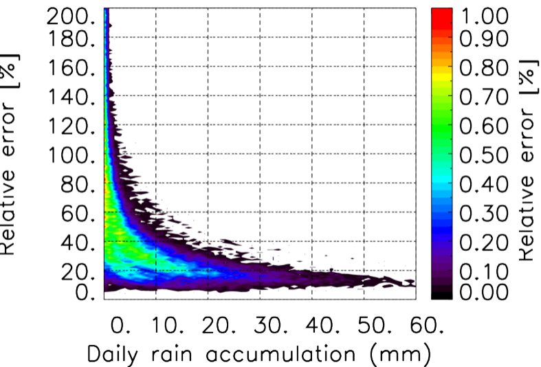
TERRE : 06 2020 00H
