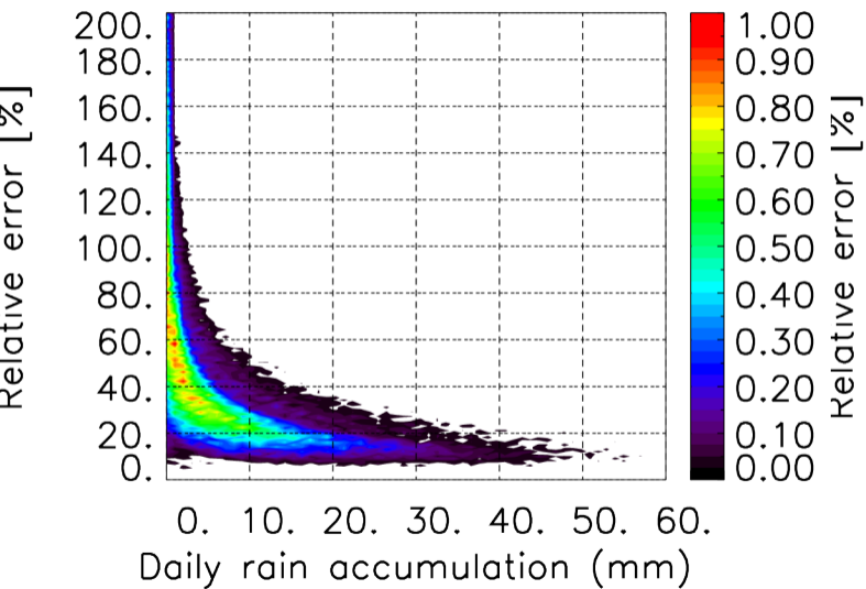
TERRE : 10 2020 00H
