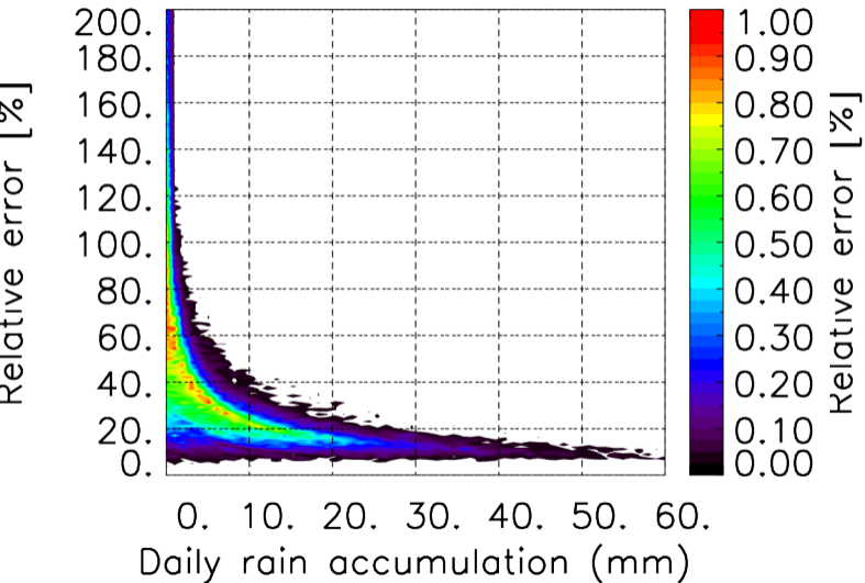
TERRE : 11 2020 00H
