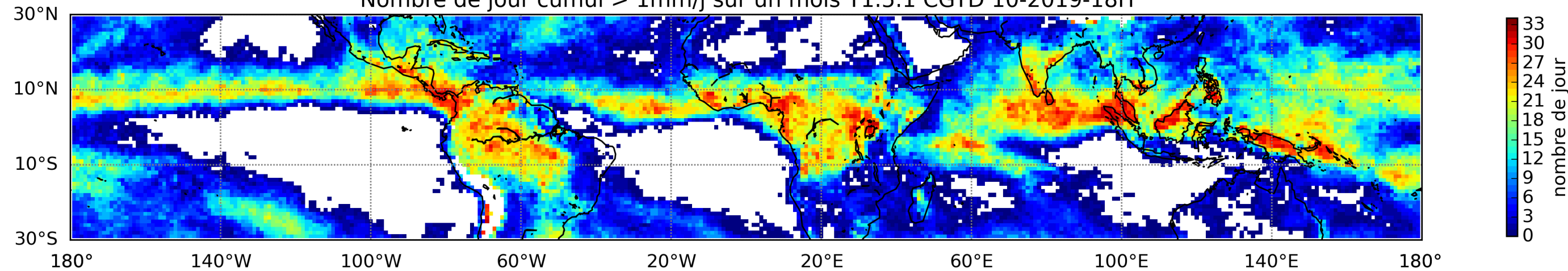
Nombre de jour cumul > 1mm/j sur un mois T1.5.1 CGTD 10-2019-18H
