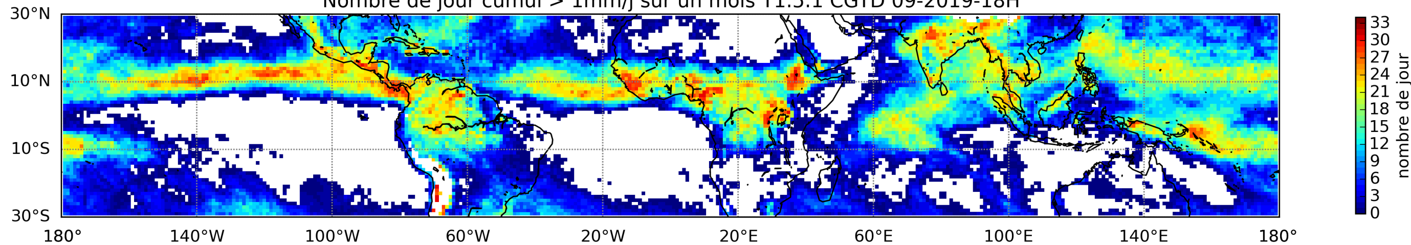
Nombre de jour cumul > 1mm/j sur un mois T1.5.1 CGTD 09-2019-18H
