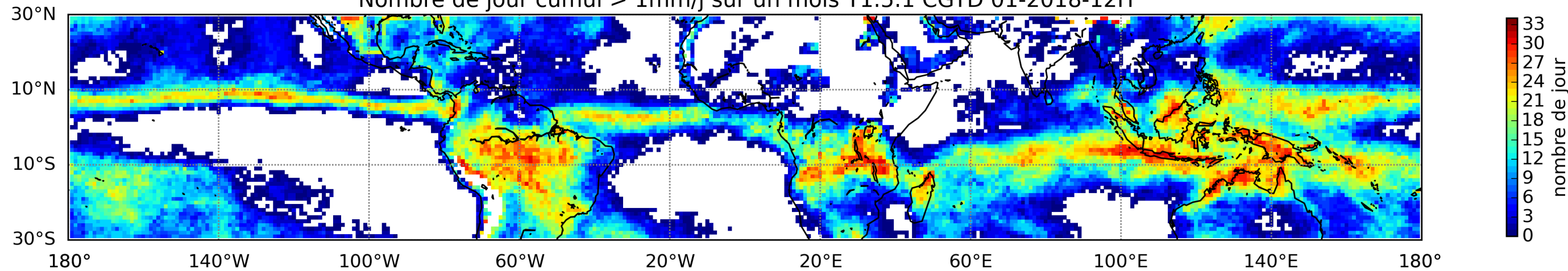
Nombre de jour cumul > 1mm/j sur un mois T1.5.1 CGTD 01-2018-12H
