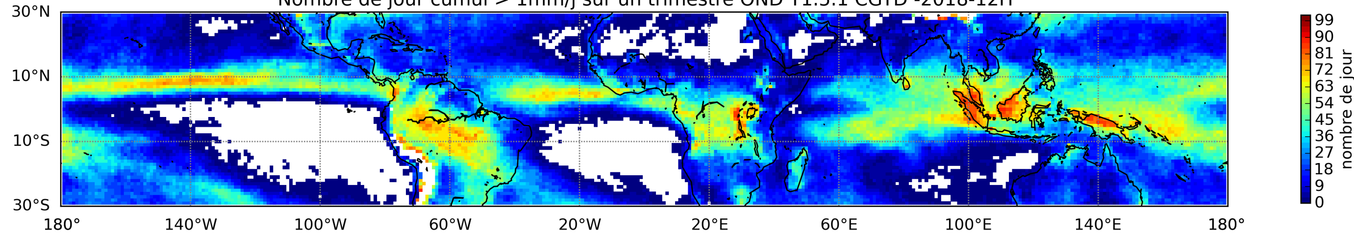
Nombre de jour cumul > 1mm/j sur un trimestre OND T1.5.1 CGTD -2018-12H
