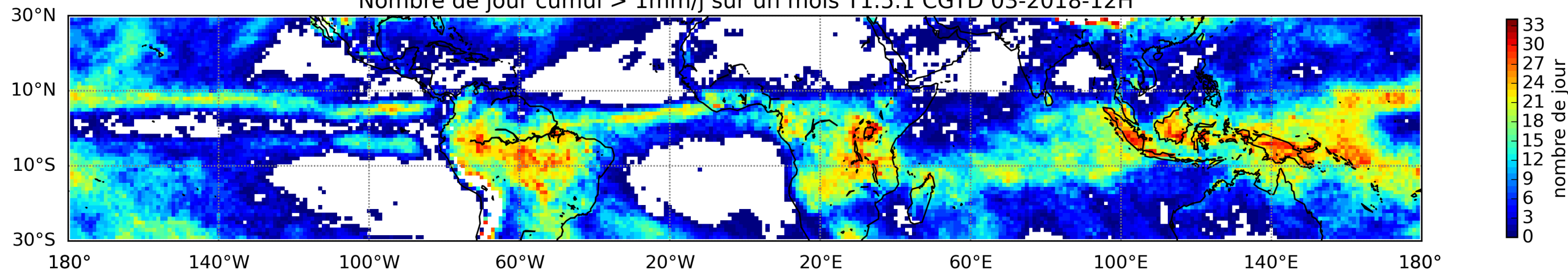
Nombre de jour cumul > 1mm/j sur un mois T1.5.1 CGTD 03-2018-12H
