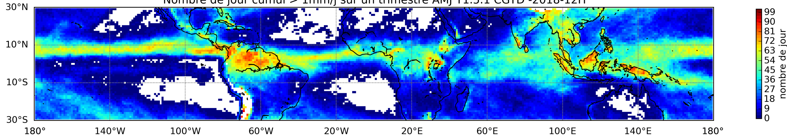
Nombre de jour cumul > 1mm/j sur un trimestre AMJ T1.5.1 CGTD -2018-12H
