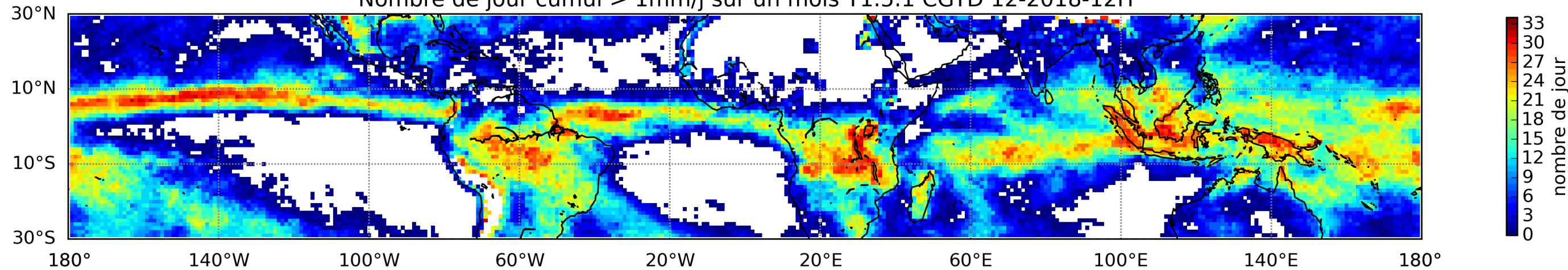
Nombre de jour cumul > 1mm/j sur un mois T1.5.1 CGTD 12-2018-12H
