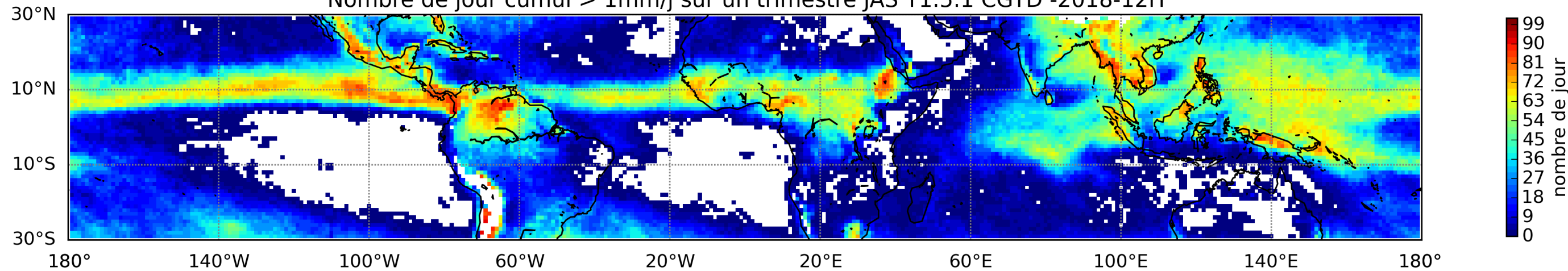
Nombre de jour cumul > 1mm/j sur un trimestre JAS T1.5.1 CGTD -2018-12H
