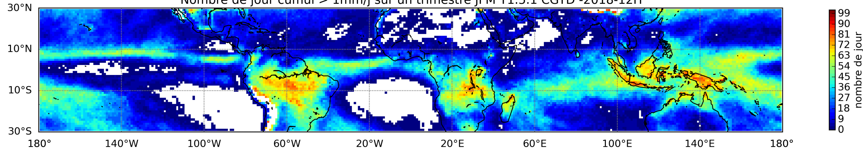
Nombre de jour cumul > 1mm/j sur un trimestre JFM T1.5.1 CGTD -2018-12H
