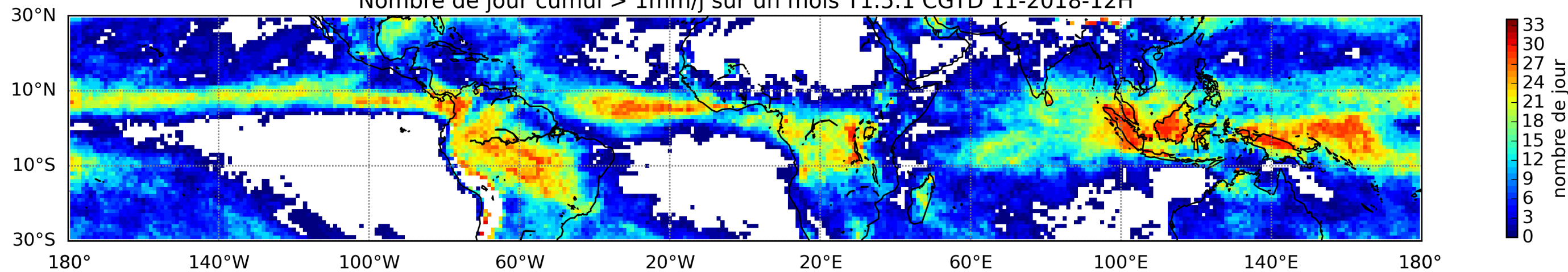
Nombre de jour cumul > 1mm/j sur un mois T1.5.1 CGTD 11-2018-12H
