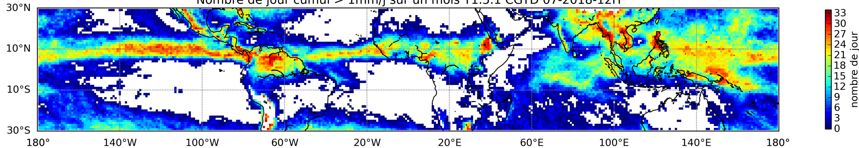
Nombre de jour cumul > 1mm/j sur un mois T1.5.1 CGTD 07-2018-12H
