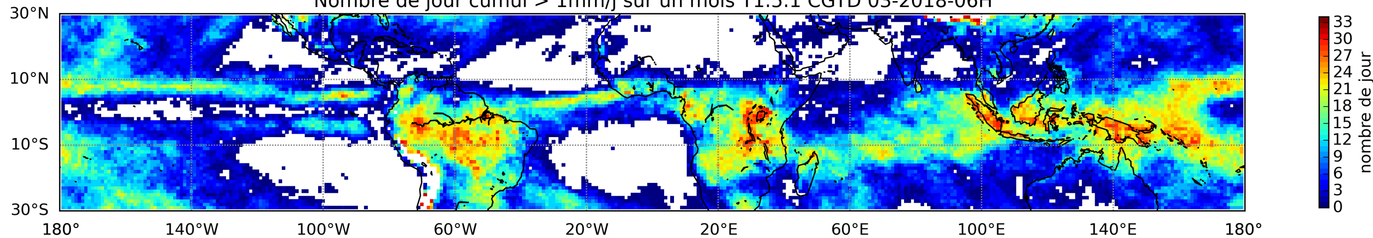
Nombre de jour cumul > 1mm/j sur un mois T1.5.1 CGTD 03-2018-06H
