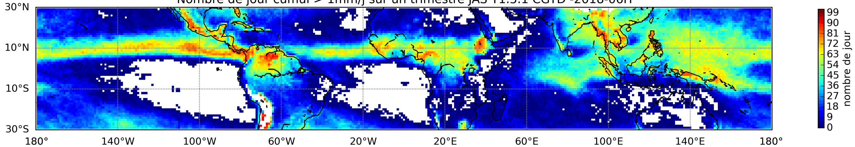
Nombre de jour cumul > 1mm/j sur un trimestre JAS T1.5.1 CGTD -2018-06H
