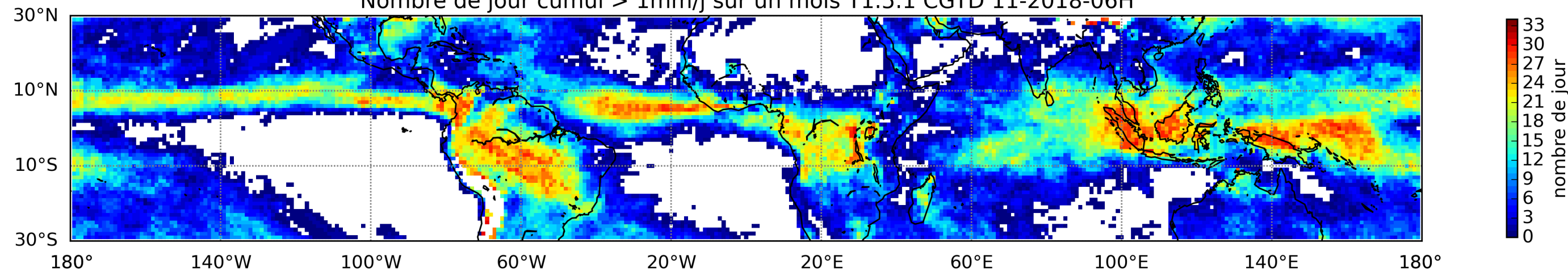
Nombre de jour cumul > 1mm/j sur un mois T1.5.1 CGTD 11-2018-06H
