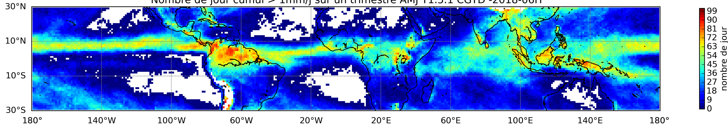
Nombre de jour cumul > 1mm/j sur un trimestre AMJ T1.5.1 CGTD -2018-06H
