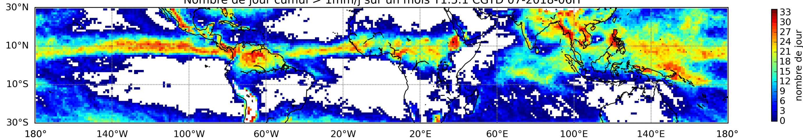
Nombre de jour cumul > 1mm/j sur un mois T1.5.1 CGTD 07-2018-06H
