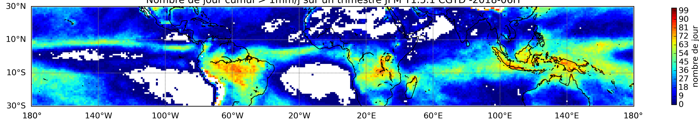
Nombre de jour cumul > 1mm/j sur un trimestre JFM T1.5.1 CGTD -2018-06H
