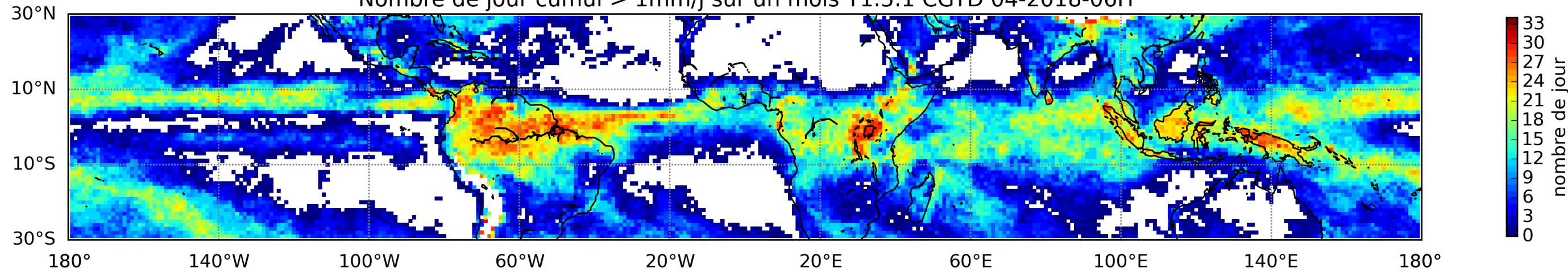
Nombre de jour cumul > 1mm/j sur un mois T1.5.1 CGTD 04-2018-06H
