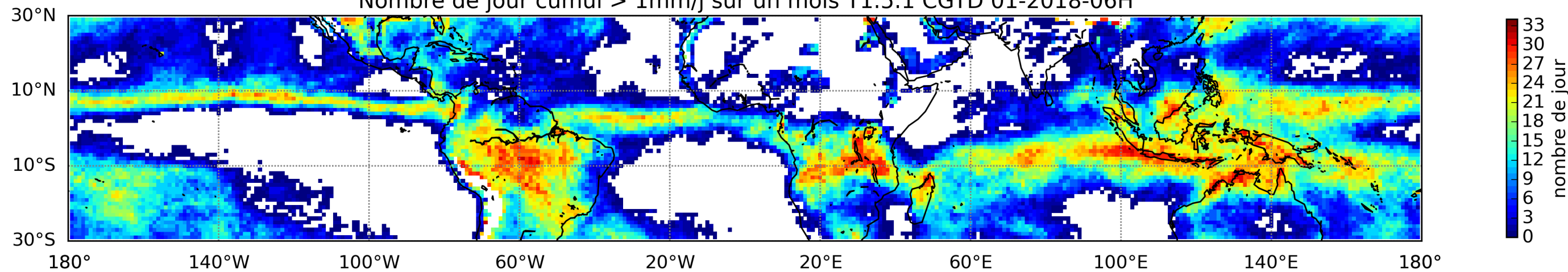
Nombre de jour cumul > 1mm/j sur un mois T1.5.1 CGTD 01-2018-06H
