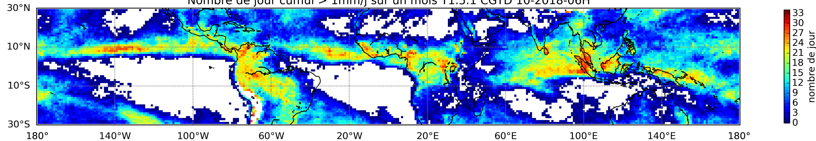
Nombre de jour cumul > 1mm/j sur un mois T1.5.1 CGTD 10-2018-06H
