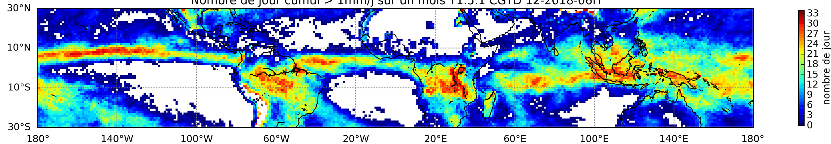
Nombre de jour cumul > 1mm/j sur un mois T1.5.1 CGTD 12-2018-06H
