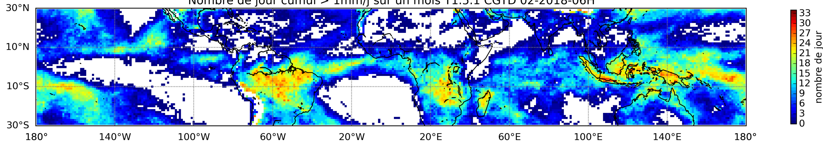
Nombre de jour cumul > 1mm/j sur un mois T1.5.1 CGTD 02-2018-06H
