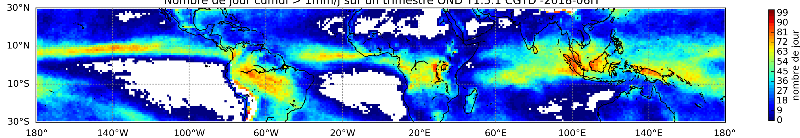
Nombre de jour cumul > 1mm/j sur un trimestre OND T1.5.1 CGTD -2018-06H
