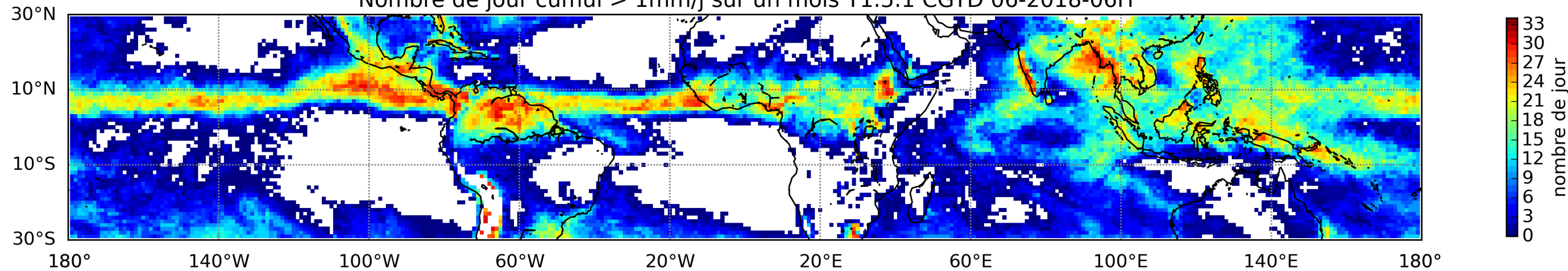
Nombre de jour cumul > 1mm/j sur un mois T1.5.1 CGTD 06-2018-06H
