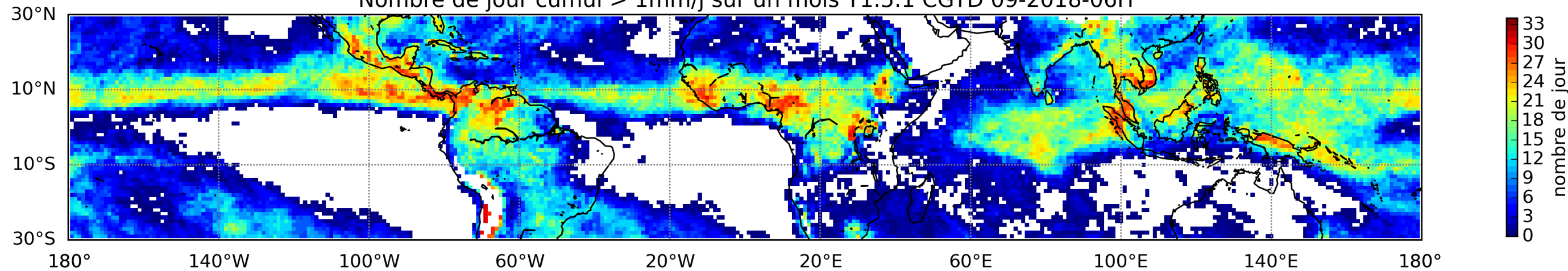
Nombre de jour cumul > 1mm/j sur un mois T1.5.1 CGTD 09-2018-06H
