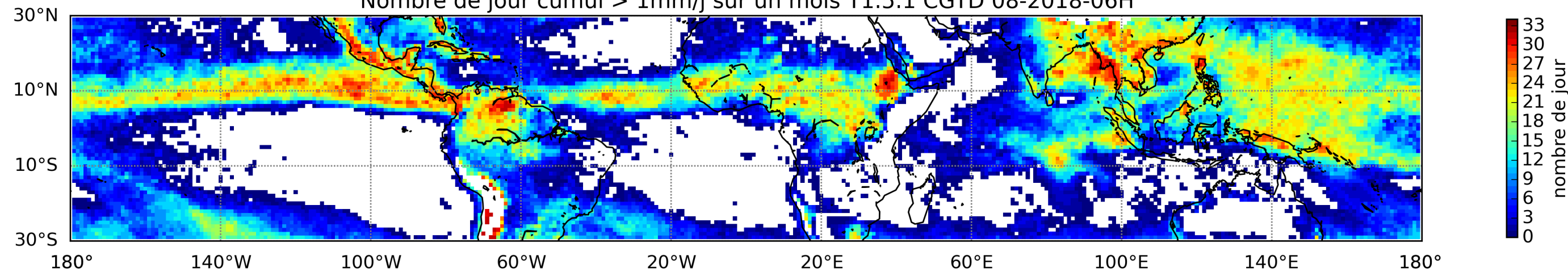
Nombre de jour cumul > 1mm/j sur un mois T1.5.1 CGTD 08-2018-06H
