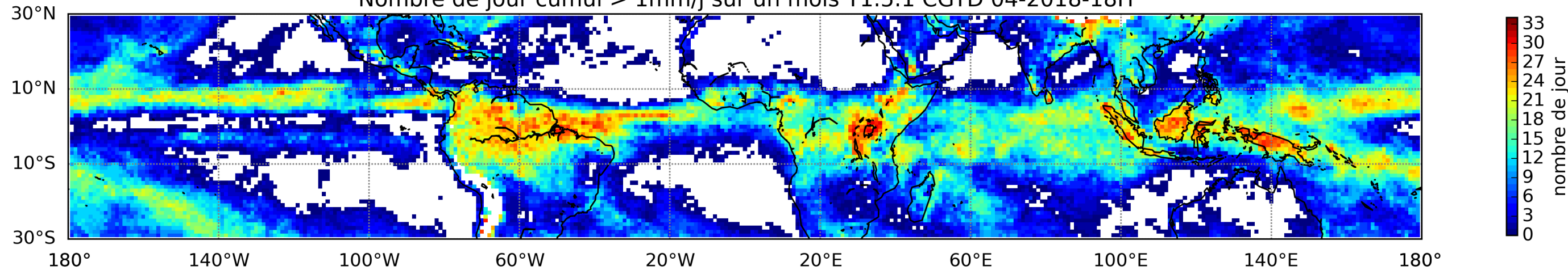
Nombre de jour cumul > 1mm/j sur un mois T1.5.1 CGTD 04-2018-18H
