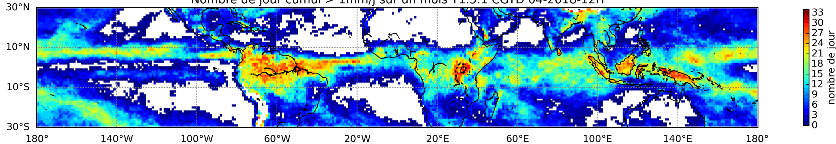
Nombre de jour cumul > 1mm/j sur un mois T1.5.1 CGTD 04-2018-12H
