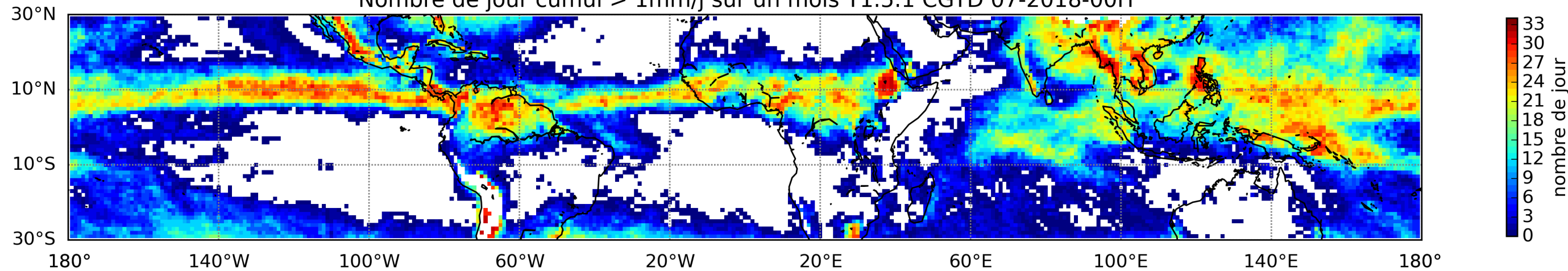
Nombre de jour cumul > 1mm/j sur un mois T1.5.1 CGTD 07-2018-00H
