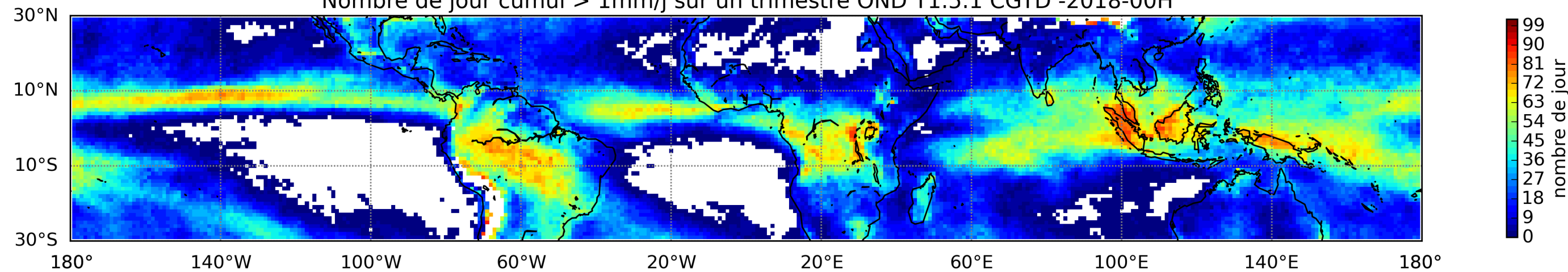
Nombre de jour cumul > 1mm/j sur un trimestre OND T1.5.1 CGTD -2018-00H
