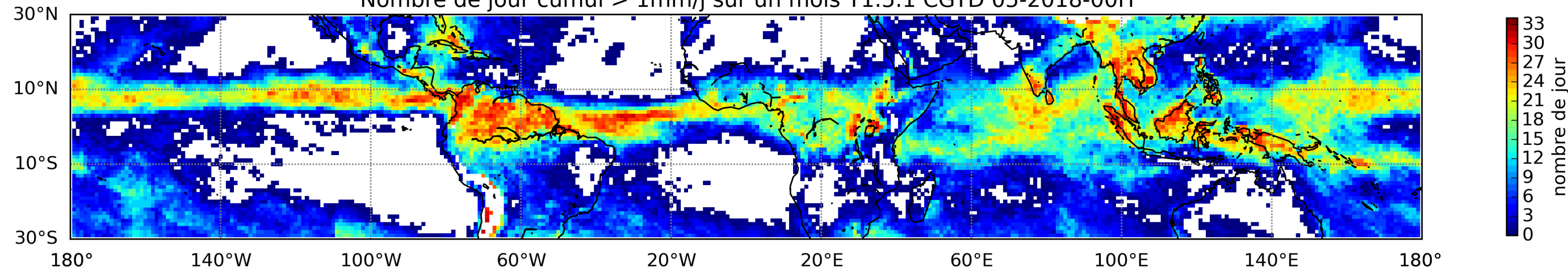
Nombre de jour cumul > 1mm/j sur un mois T1.5.1 CGTD 05-2018-00H
