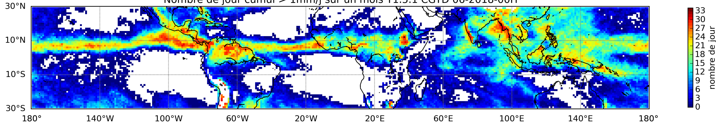
Nombre de jour cumul > 1mm/j sur un mois T1.5.1 CGTD 06-2018-00H
