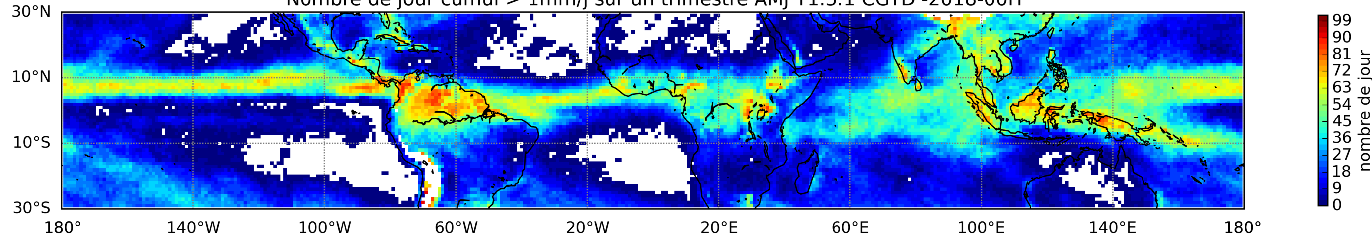
Nombre de jour cumul > 1mm/j sur un trimestre AMJ T1.5.1 CGTD -2018-00H
