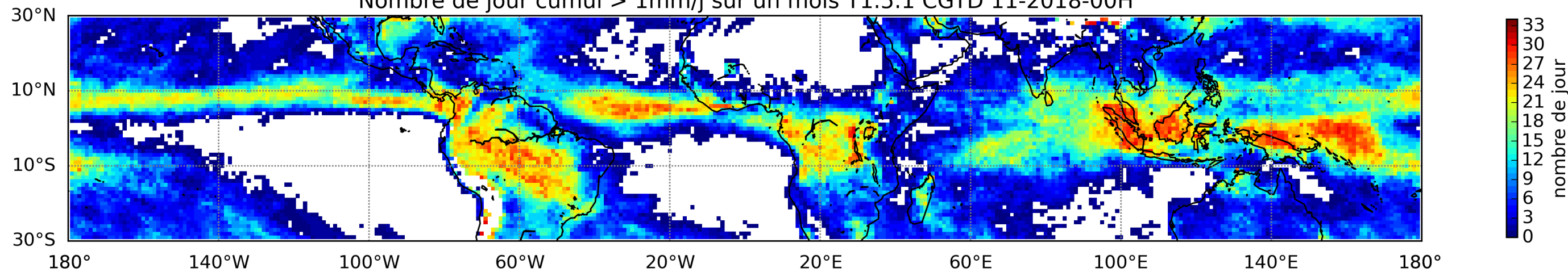
Nombre de jour cumul > 1mm/j sur un mois T1.5.1 CGTD 11-2018-00H
