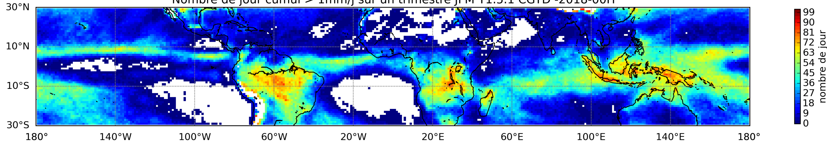
Nombre de jour cumul > 1mm/j sur un trimestre JFM T1.5.1 CGTD -2018-00H
