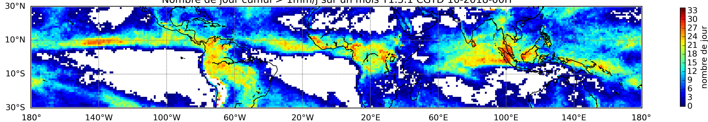
Nombre de jour cumul > 1mm/j sur un mois T1.5.1 CGTD 10-2018-00H
