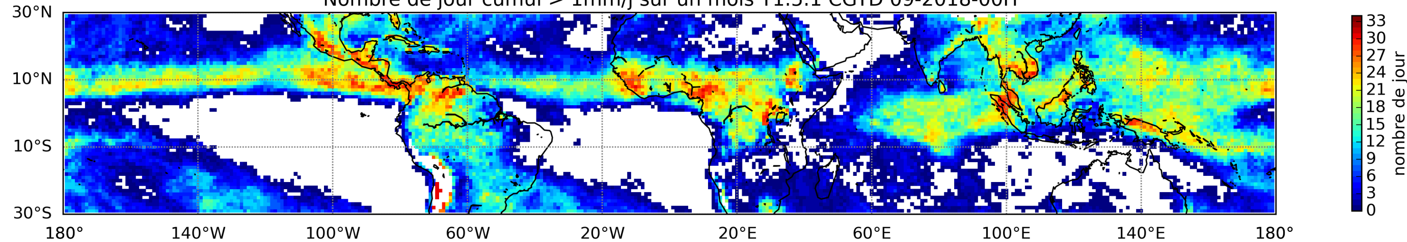
Nombre de jour cumul > 1mm/j sur un mois T1.5.1 CGTD 09-2018-00H
