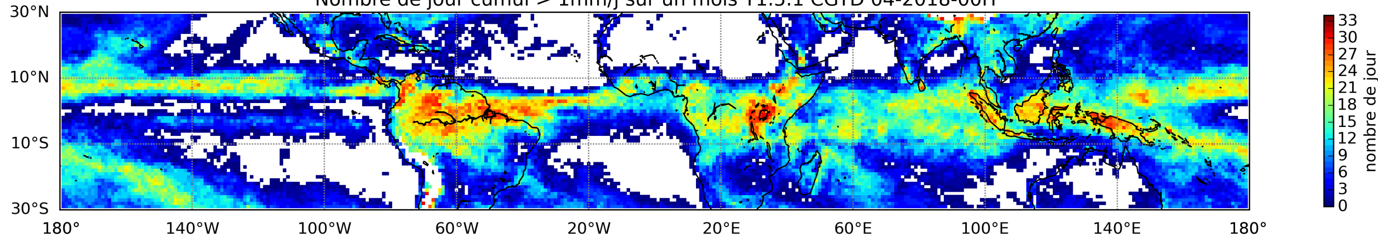
Nombre de jour cumul > 1mm/j sur un mois T1.5.1 CGTD 04-2018-00H
