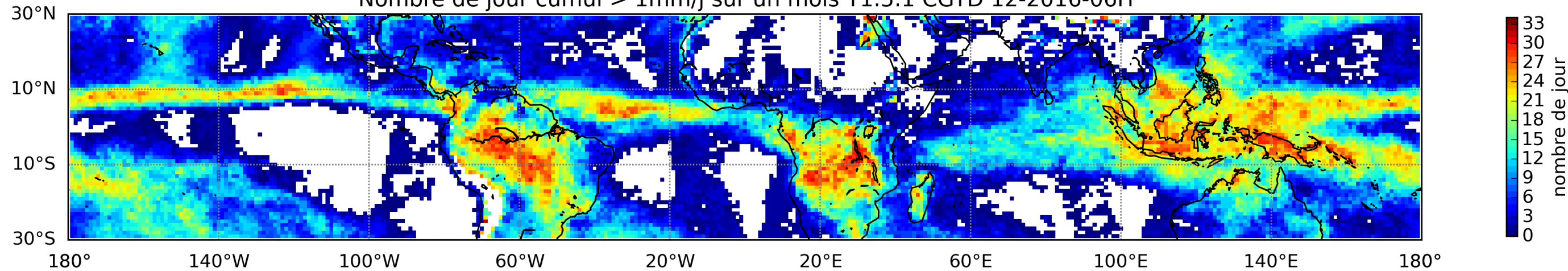
Nombre de jour cumul > 1mm/j sur un mois T1.5.1 CGTD 12-2016-06H
