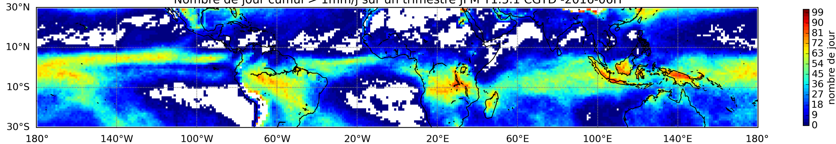
Nombre de jour cumul > 1mm/j sur un trimestre JFM T1.5.1 CGTD -2016-06H
