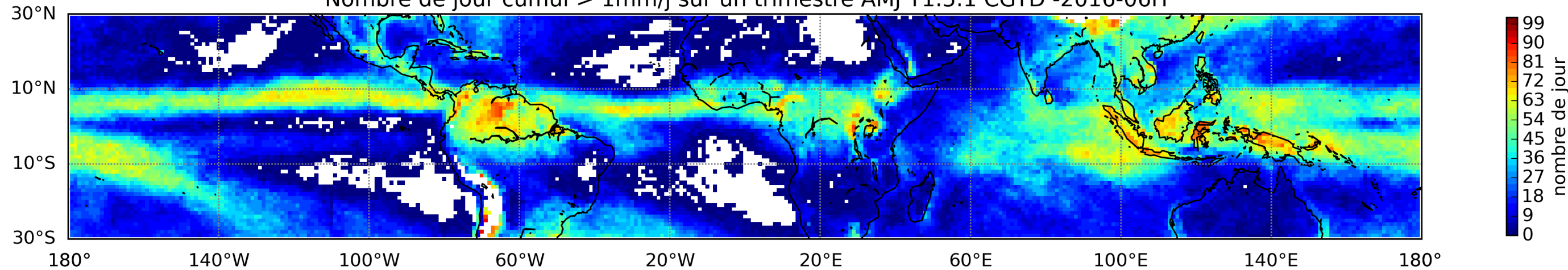
Nombre de jour cumul > 1mm/j sur un trimestre AMJ T1.5.1 CGTD -2016-06H
