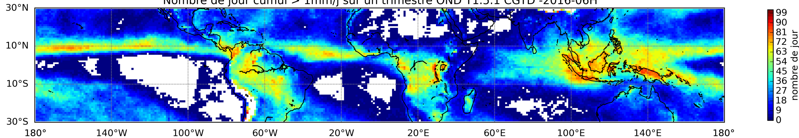
Nombre de jour cumul > 1mm/j sur un trimestre OND T1.5.1 CGTD -2016-06H
