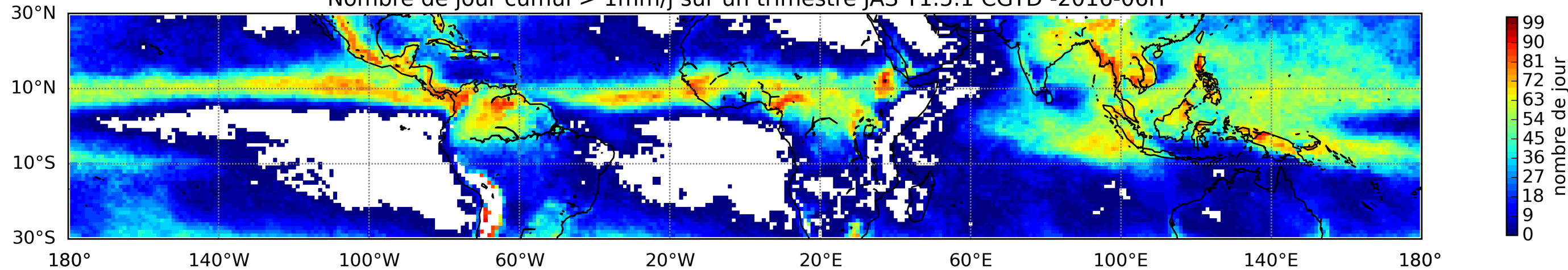
Nombre de jour cumul > 1mm/j sur un trimestre JAS T1.5.1 CGTD -2016-06H
