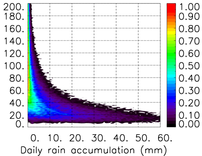
MER : 05 2016 06H
