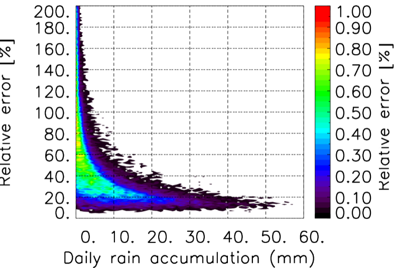
TERRE : 05 2016 06H
