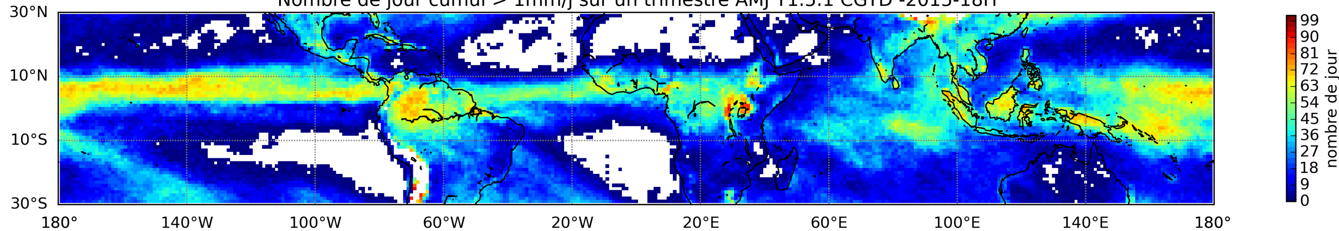
Nombre de jour cumul > 1mm/j sur un trimestre AMJ T1.5.1 CGTD -2015-18H
