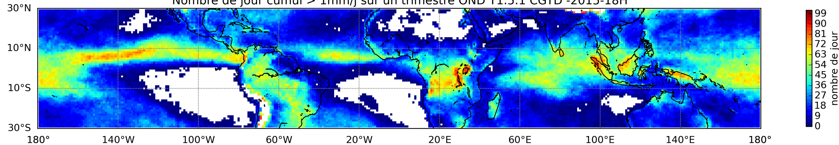
Nombre de jour cumul > 1mm/j sur un trimestre OND T1.5.1 CGTD -2015-18H
