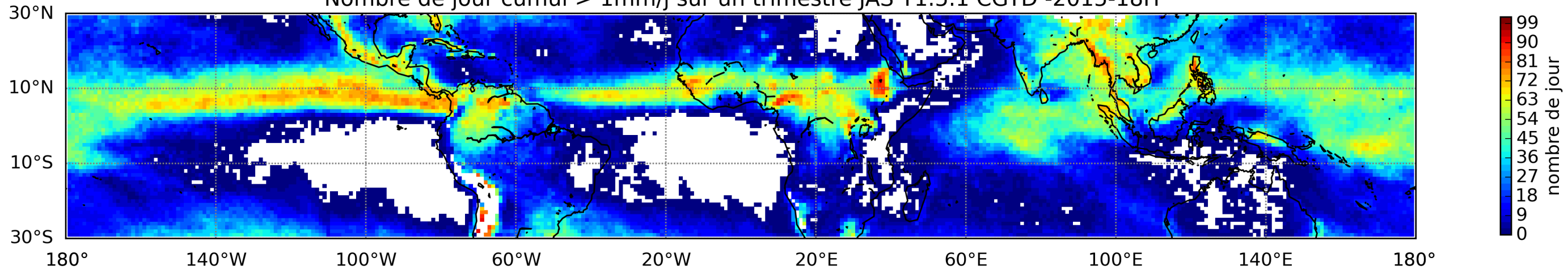
Nombre de jour cumul > 1mm/j sur un trimestre JAS T1.5.1 CGTD -2015-18H
