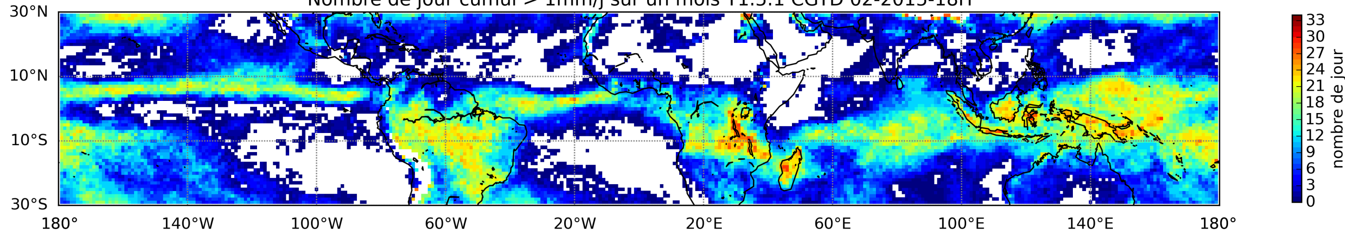
Nombre de jour cumul > 1mm/j sur un mois T1.5.1 CGTD 02-2015-18H
