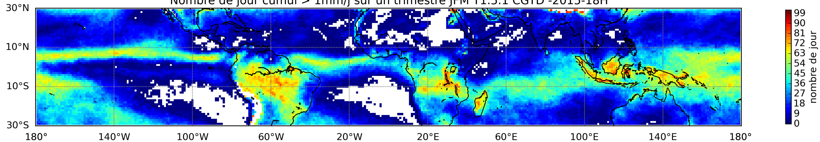
Nombre de jour cumul > 1mm/j sur un trimestre JFM T1.5.1 CGTD -2015-18H
