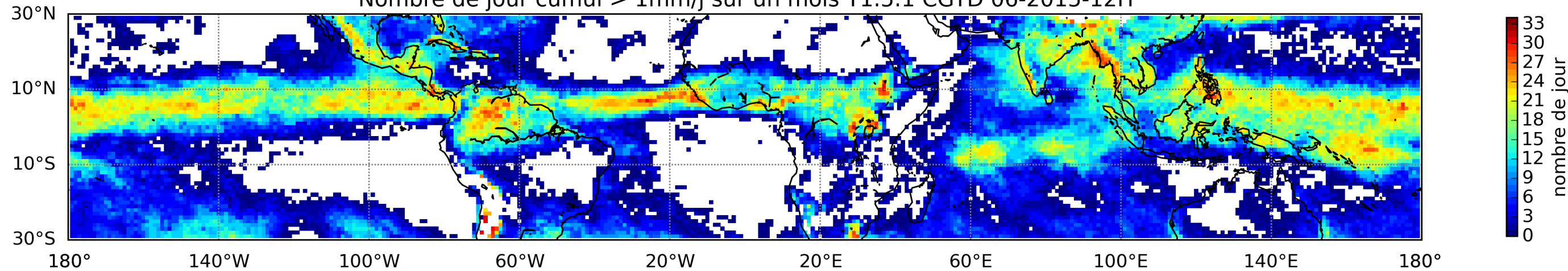
Nombre de jour cumul > 1mm/j sur un mois T1.5.1 CGTD 06-2015-12H
