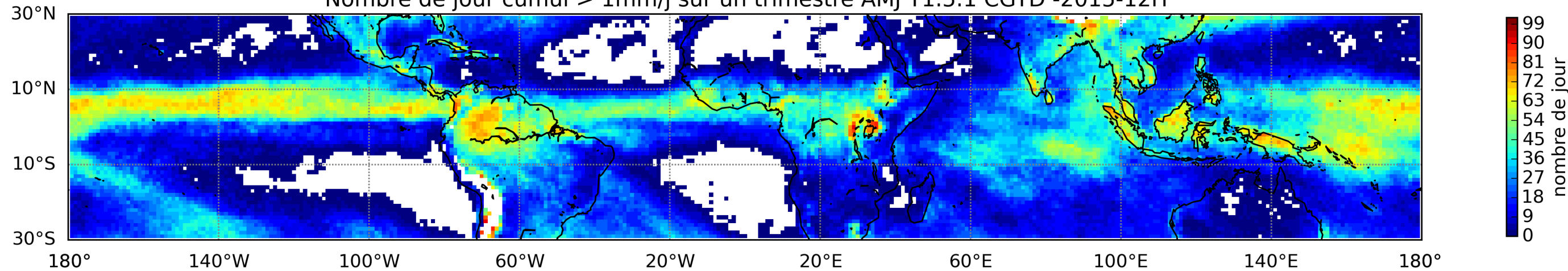
Nombre de jour cumul > 1mm/j sur un trimestre AMJ T1.5.1 CGTD -2015-12H
