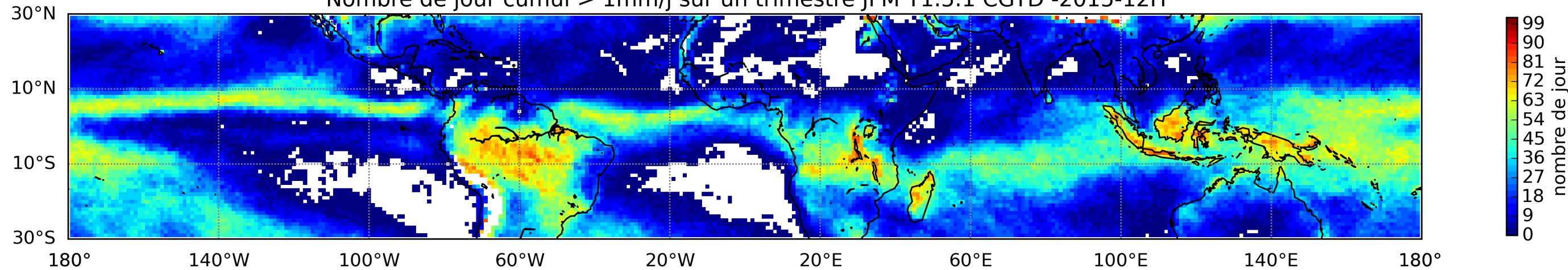
Nombre de jour cumul > 1mm/j sur un trimestre JFM T1.5.1 CGTD -2015-12H
