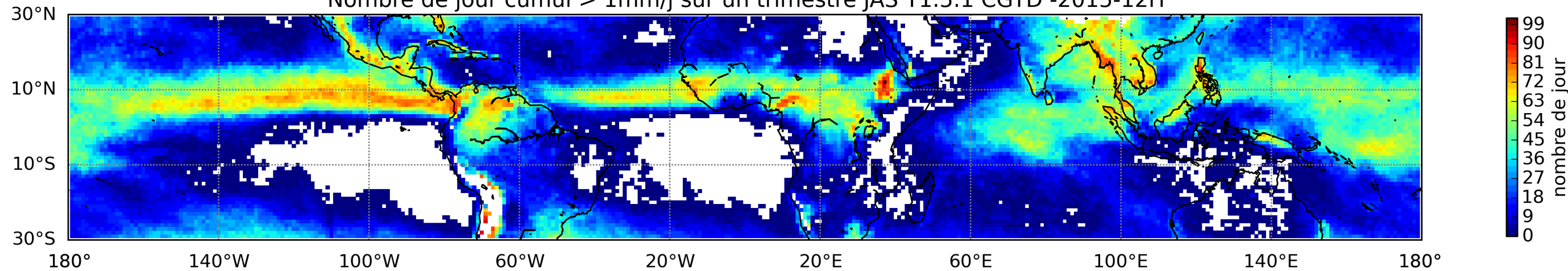
Nombre de jour cumul > 1mm/j sur un trimestre JAS T1.5.1 CGTD -2015-12H
