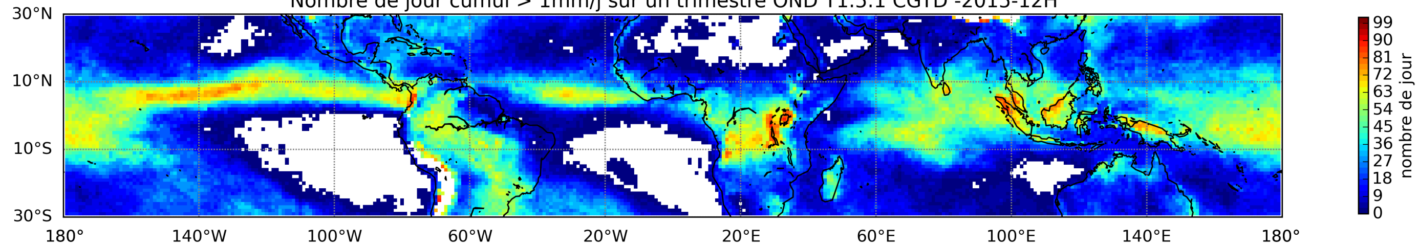
Nombre de jour cumul > 1mm/j sur un trimestre OND T1.5.1 CGTD -2015-12H
