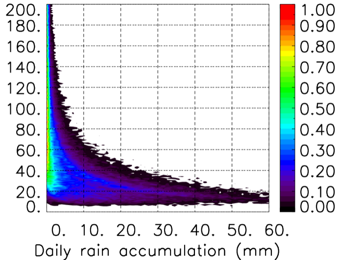
MER : 10 2015 12H
