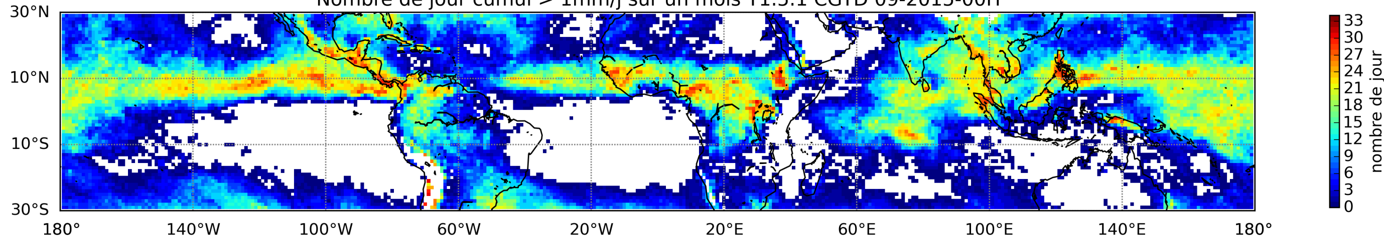
Nombre de jour cumul > 1mm/j sur un mois T1.5.1 CGTD 09-2015-00H
