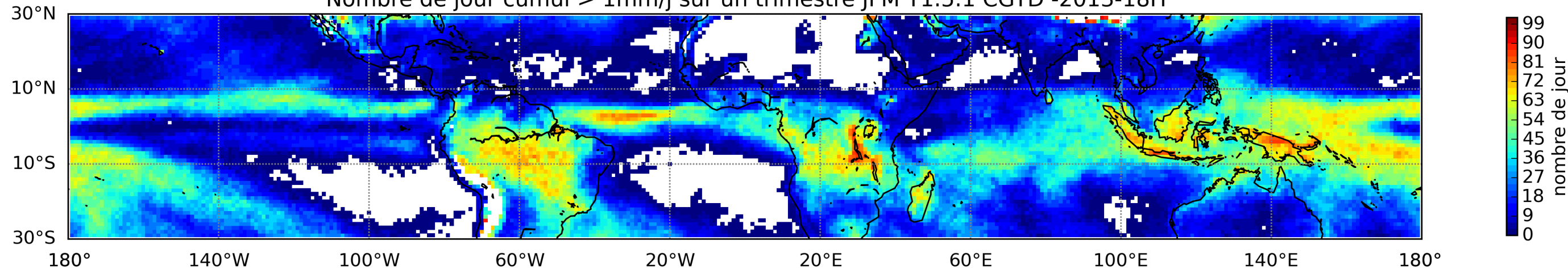
Nombre de jour cumul > 1mm/j sur un trimestre JFM T1.5.1 CGTD -2013-18H
