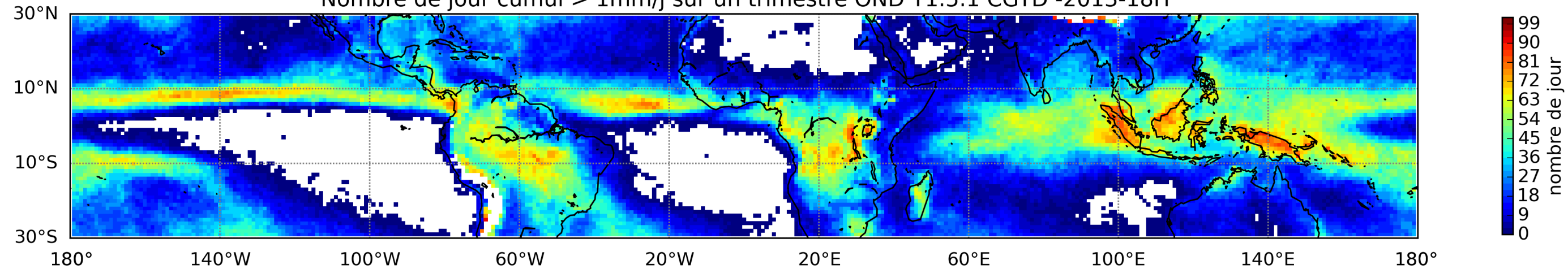
Nombre de jour cumul > 1mm/j sur un trimestre OND T1.5.1 CGTD -2013-18H
