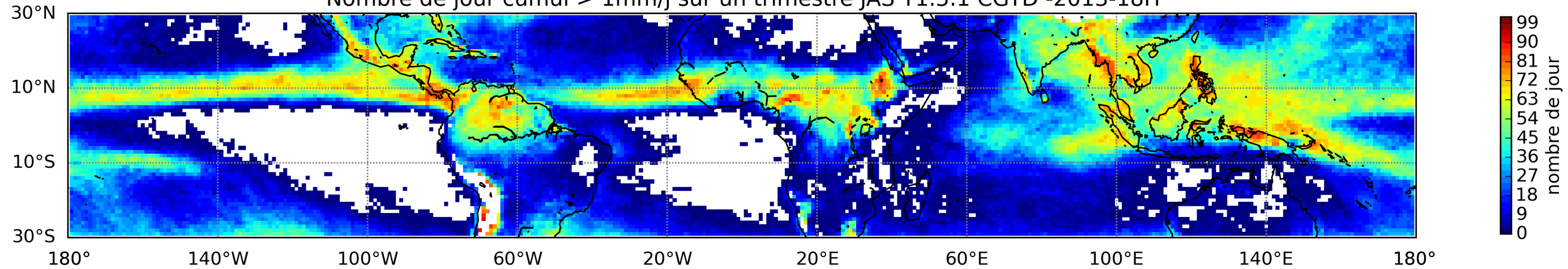
Nombre de jour cumul > 1mm/j sur un trimestre JAS T1.5.1 CGTD -2013-18H
