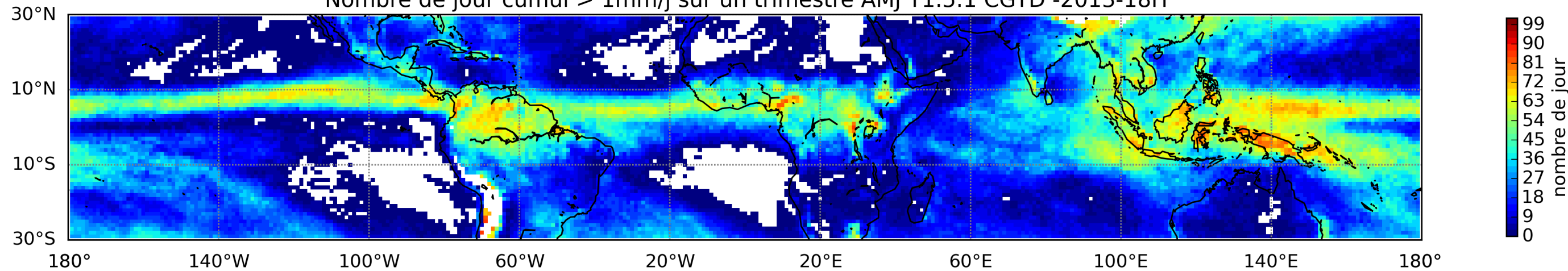
Nombre de jour cumul > 1mm/j sur un trimestre AMJ T1.5.1 CGTD -2013-18H
