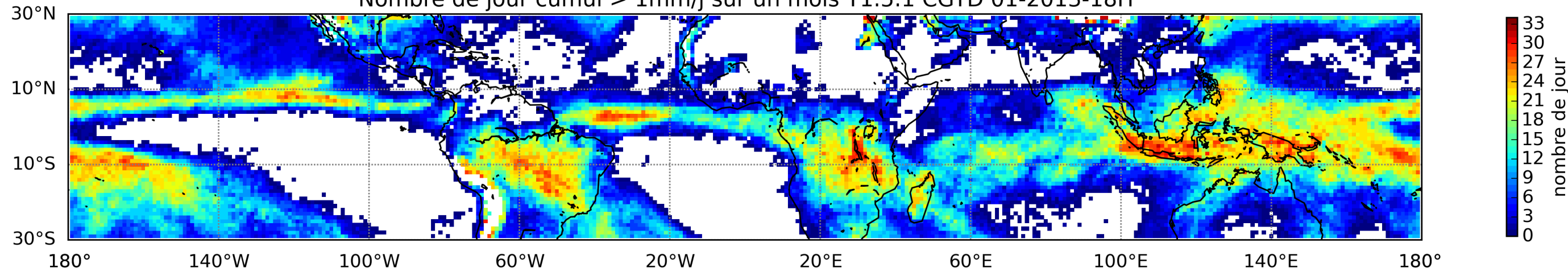
Nombre de jour cumul > 1mm/j sur un mois T1.5.1 CGTD 01-2013-18H
