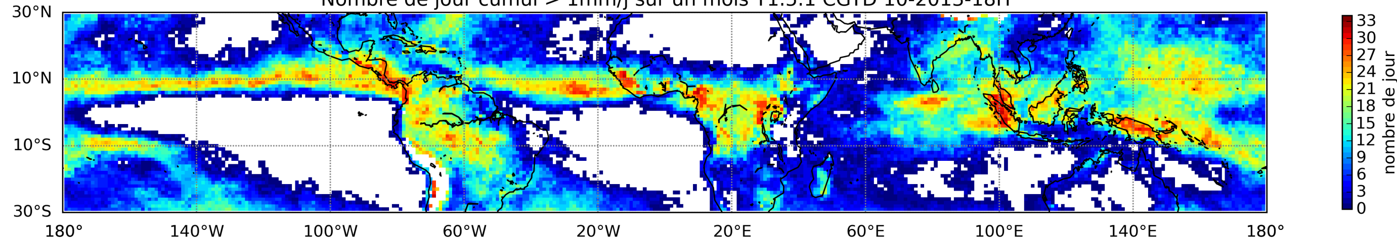
Nombre de jour cumul > 1mm/j sur un mois T1.5.1 CGTD 10-2013-18H
