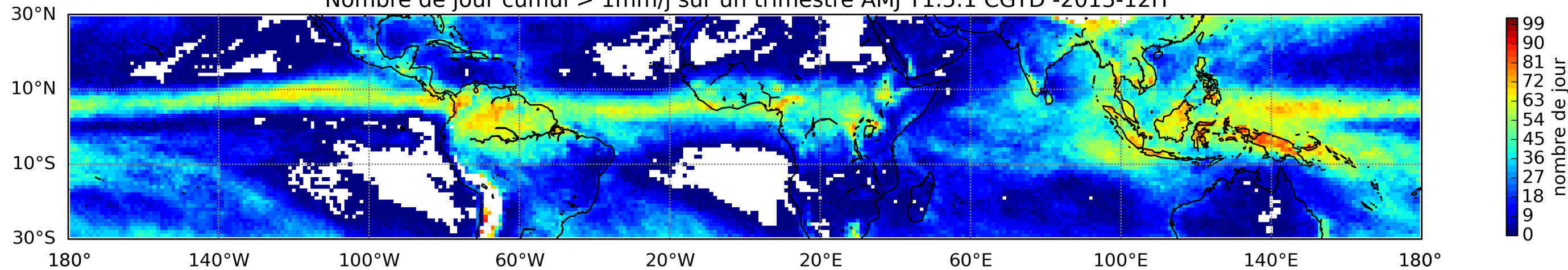
Nombre de jour cumul > 1mm/j sur un trimestre AMJ T1.5.1 CGTD -2013-12H
