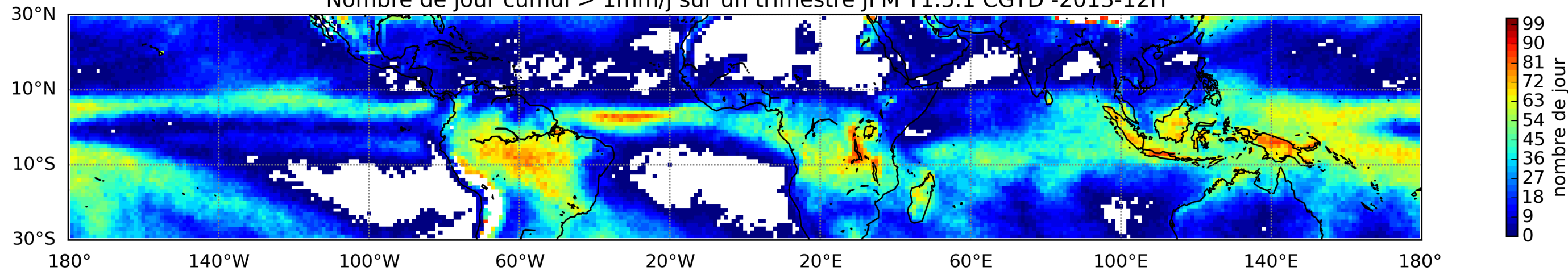
Nombre de jour cumul > 1mm/j sur un trimestre JFM T1.5.1 CGTD -2013-12H
