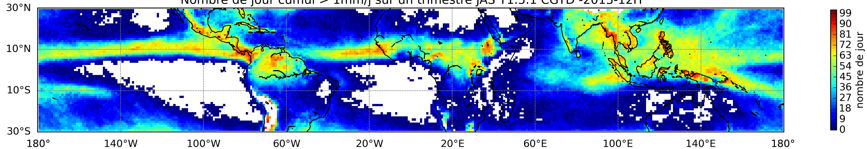
Nombre de jour cumul > 1mm/j sur un trimestre JAS T1.5.1 CGTD -2013-12H
