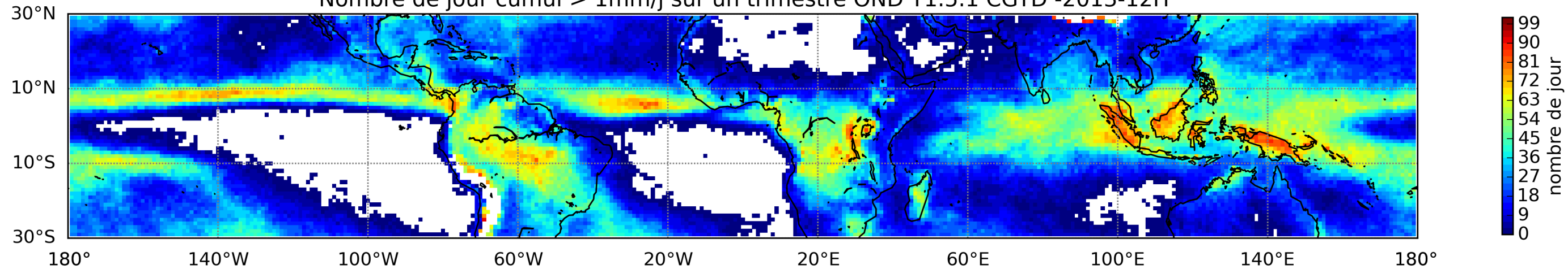
Nombre de jour cumul > 1mm/j sur un trimestre OND T1.5.1 CGTD -2013-12H
