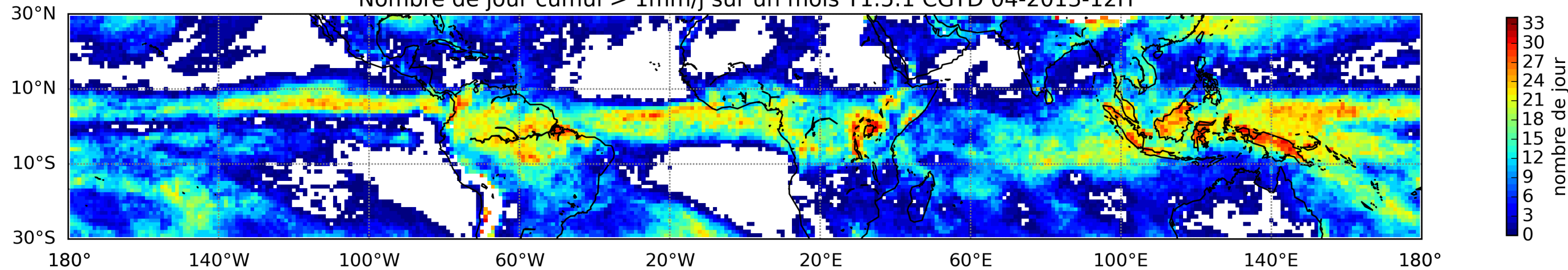
Nombre de jour cumul > 1mm/j sur un mois T1.5.1 CGTD 04-2013-12H
