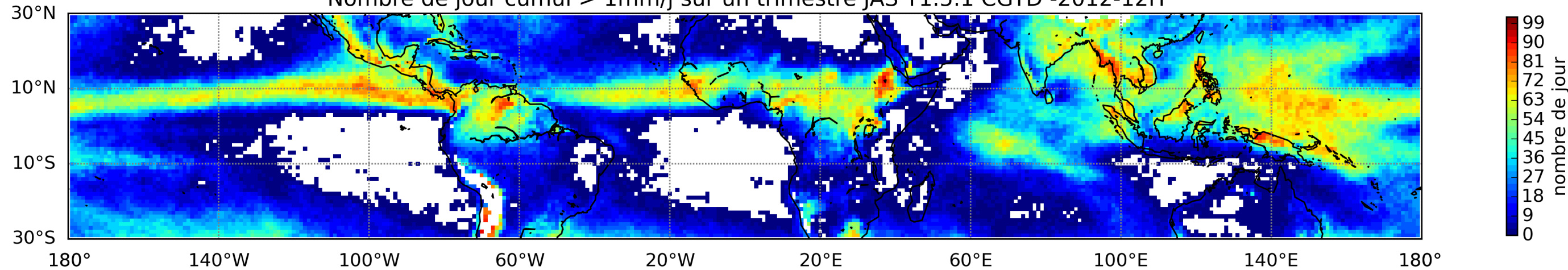
Nombre de jour cumul > 1mm/j sur un trimestre JAS T1.5.1 CGTD -2012-12H
