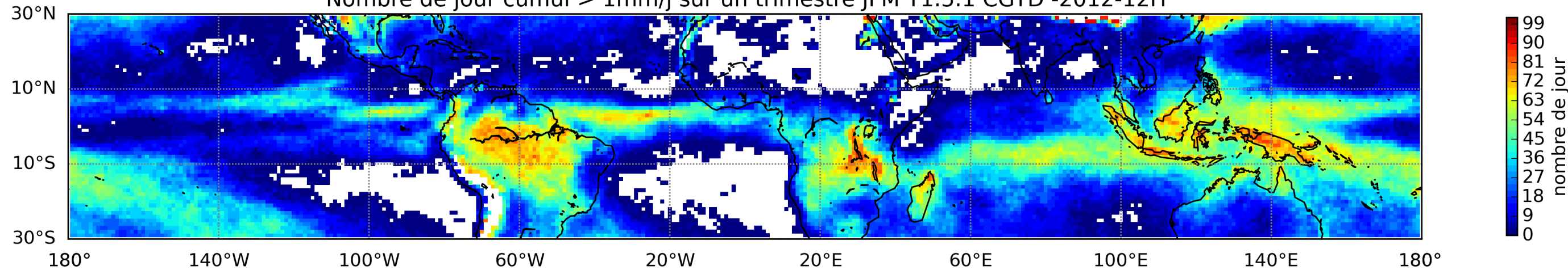
Nombre de jour cumul > 1mm/j sur un trimestre JFM T1.5.1 CGTD -2012-12H
