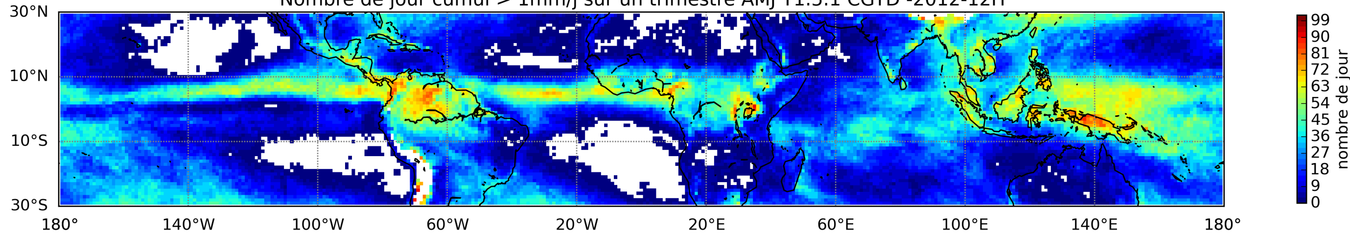
Nombre de jour cumul > 1mm/j sur un trimestre AMJ T1.5.1 CGTD -2012-12H
