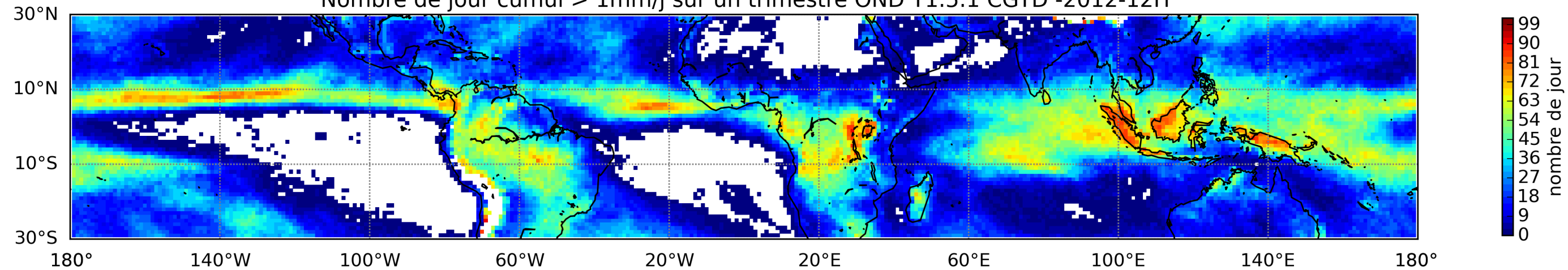
Nombre de jour cumul > 1mm/j sur un trimestre OND T1.5.1 CGTD -2012-12H
