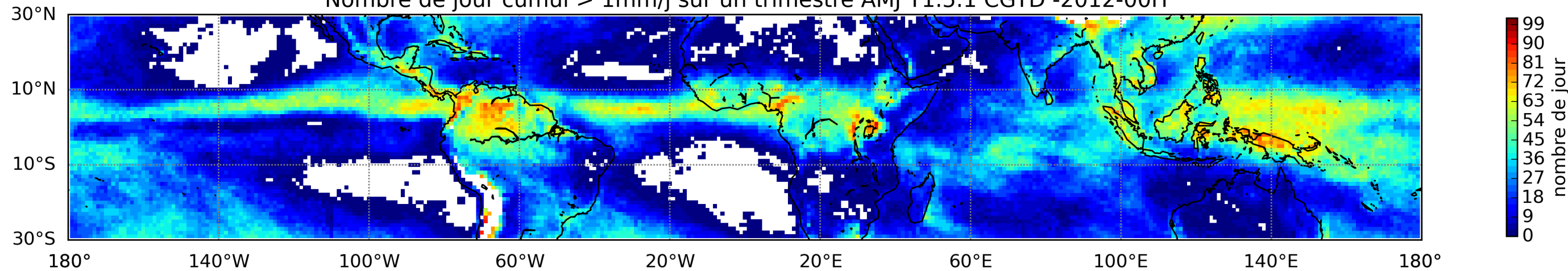
Nombre de jour cumul > 1mm/j sur un trimestre AMJ T1.5.1 CGTD -2012-00H
