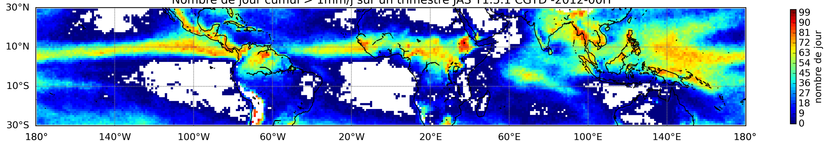
Nombre de jour cumul > 1mm/j sur un trimestre JAS T1.5.1 CGTD -2012-00H
