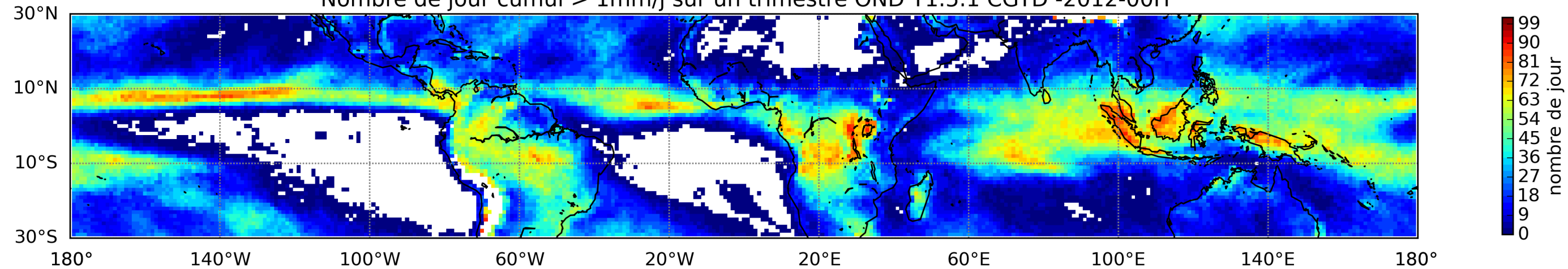
Nombre de jour cumul > 1mm/j sur un trimestre OND T1.5.1 CGTD -2012-00H
