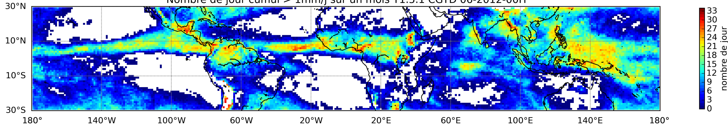
Nombre de jour cumul > 1mm/j sur un mois T1.5.1 CGTD 06-2012-00H
