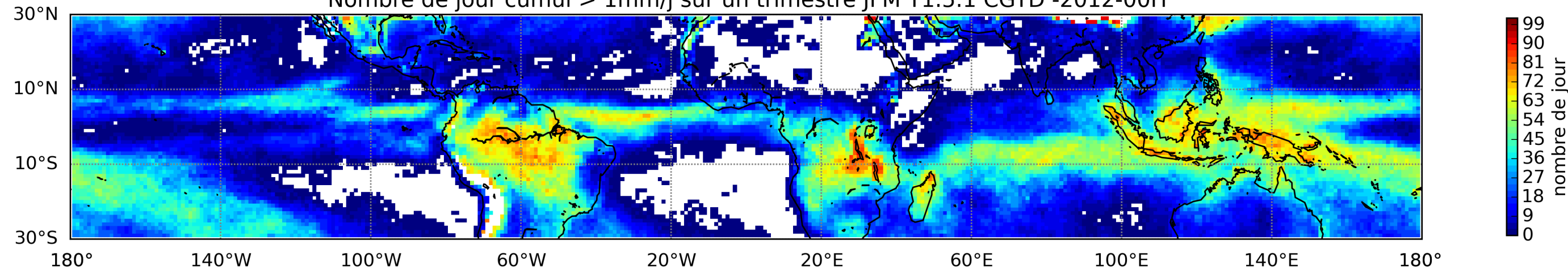
Nombre de jour cumul > 1mm/j sur un trimestre JFM T1.5.1 CGTD -2012-00H
