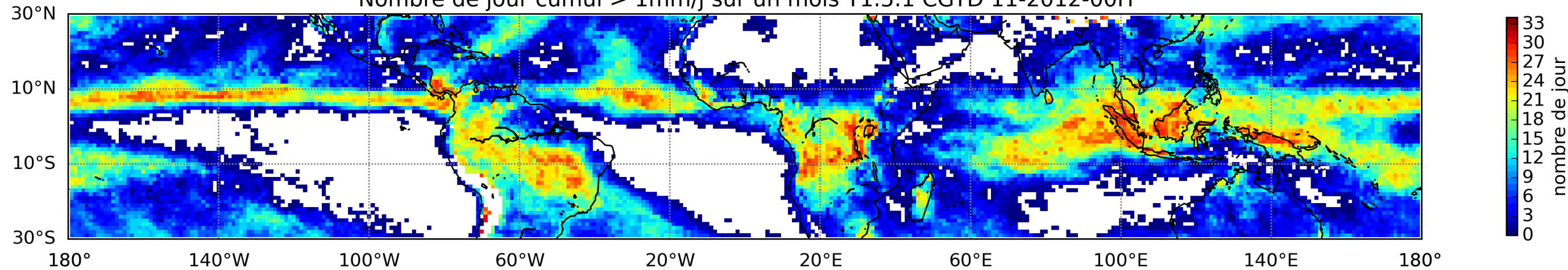
Nombre de jour cumul > 1mm/j sur un mois T1.5.1 CGTD 11-2012-00H
