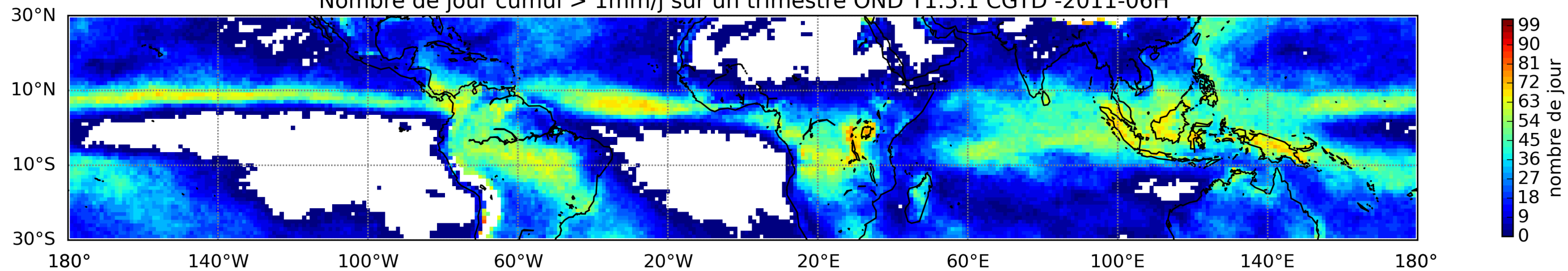
Nombre de jour cumul > 1mm/j sur un trimestre OND T1.5.1 CGTD -2011-06H
