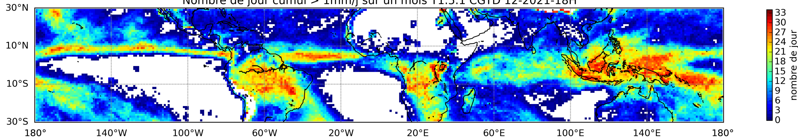
Nombre de jour cumul > 1mm/j sur un mois T1.5.1 CGTD 12-2021-18H
