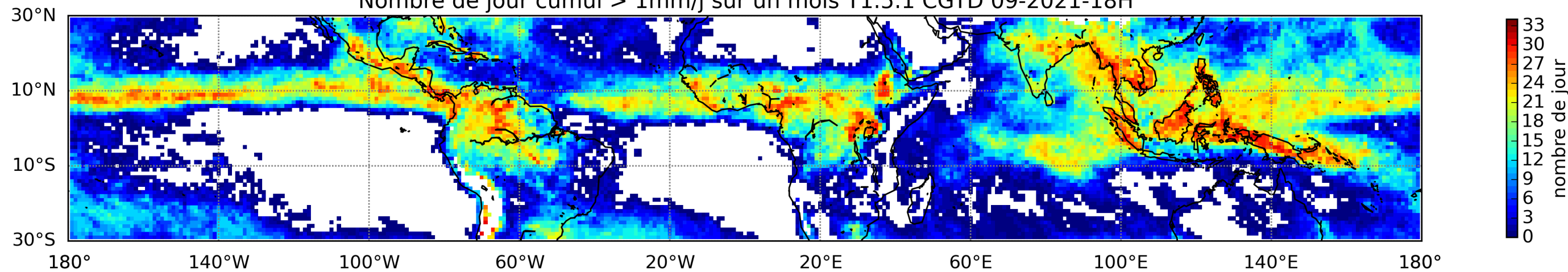
Nombre de jour cumul > 1mm/j sur un mois T1.5.1 CGTD 09-2021-18H
