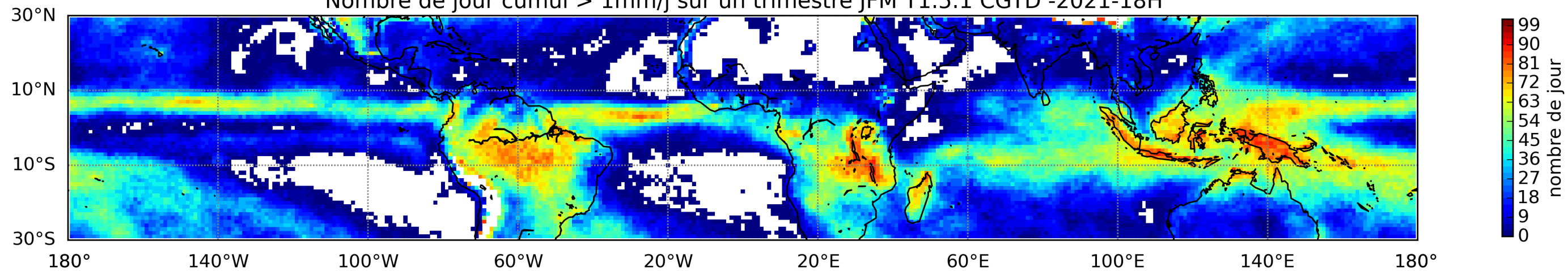
Nombre de jour cumul > 1mm/j sur un trimestre JFM T1.5.1 CGTD -2021-18H
