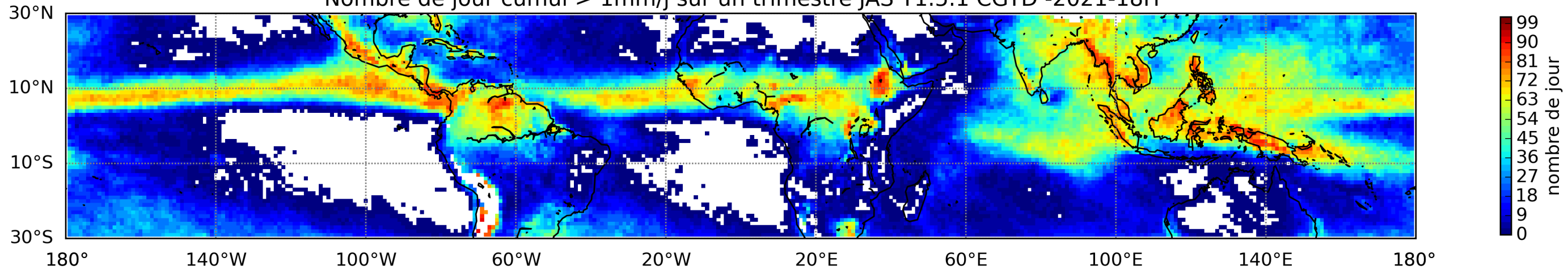
Nombre de jour cumul > 1mm/j sur un trimestre JAS T1.5.1 CGTD -2021-18H
