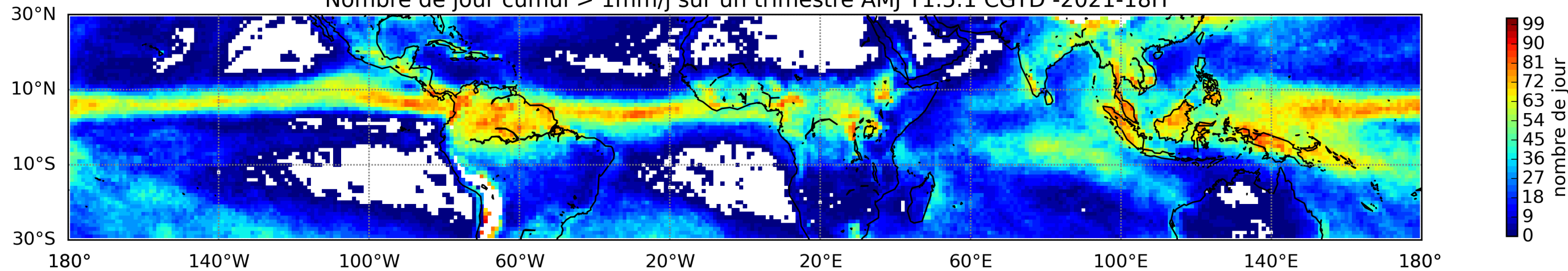
Nombre de jour cumul > 1mm/j sur un trimestre AMJ T1.5.1 CGTD -2021-18H
