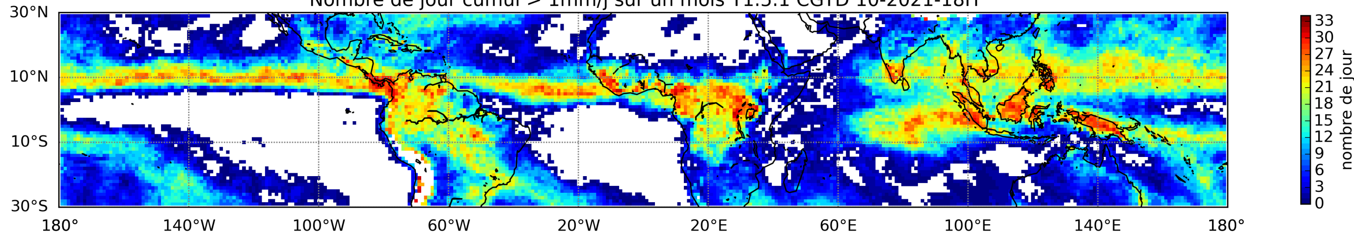
Nombre de jour cumul > 1mm/j sur un mois T1.5.1 CGTD 10-2021-18H
