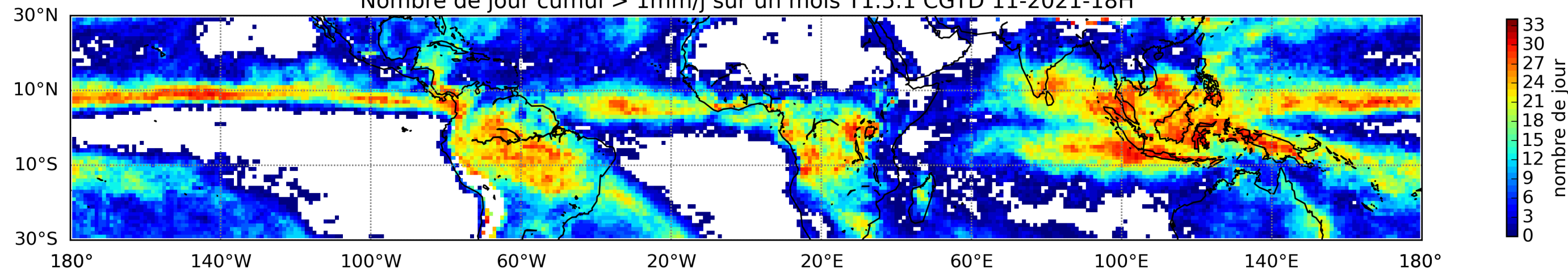
Nombre de jour cumul > 1mm/j sur un mois T1.5.1 CGTD 11-2021-18H
