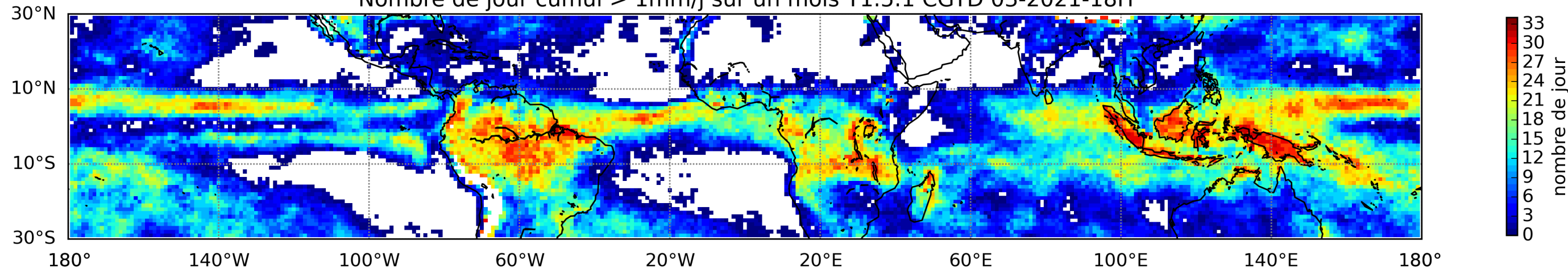
Nombre de jour cumul > 1mm/j sur un mois T1.5.1 CGTD 03-2021-18H
