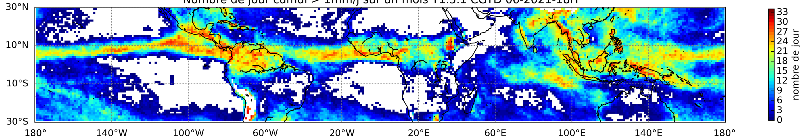
Nombre de jour cumul > 1mm/j sur un mois T1.5.1 CGTD 06-2021-18H
