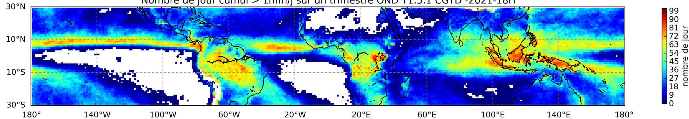
Nombre de jour cumul > 1mm/j sur un trimestre OND T1.5.1 CGTD -2021-18H
