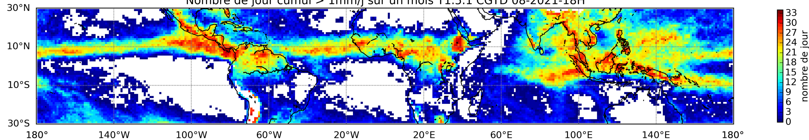
Nombre de jour cumul > 1mm/j sur un mois T1.5.1 CGTD 08-2021-18H
