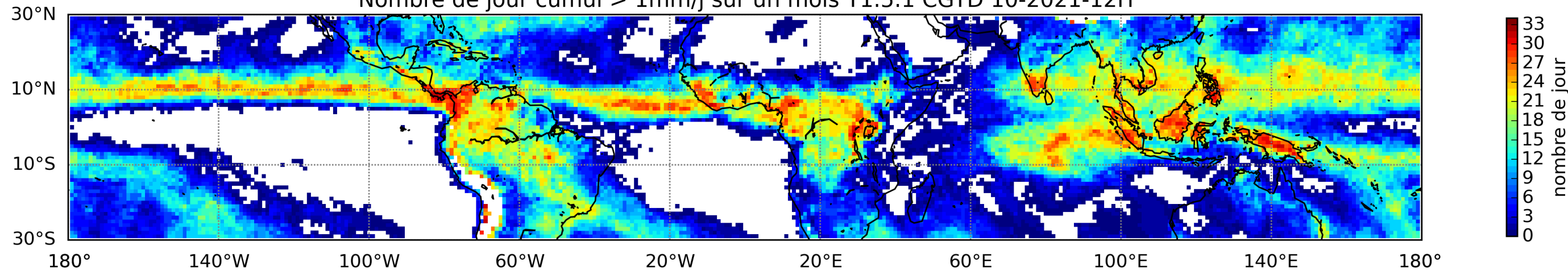
Nombre de jour cumul > 1mm/j sur un mois T1.5.1 CGTD 10-2021-12H
