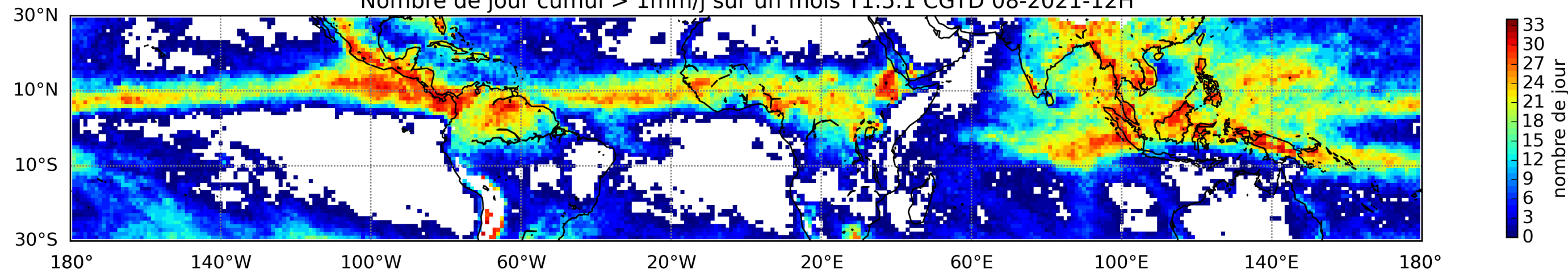
Nombre de jour cumul > 1mm/j sur un mois T1.5.1 CGTD 08-2021-12H
