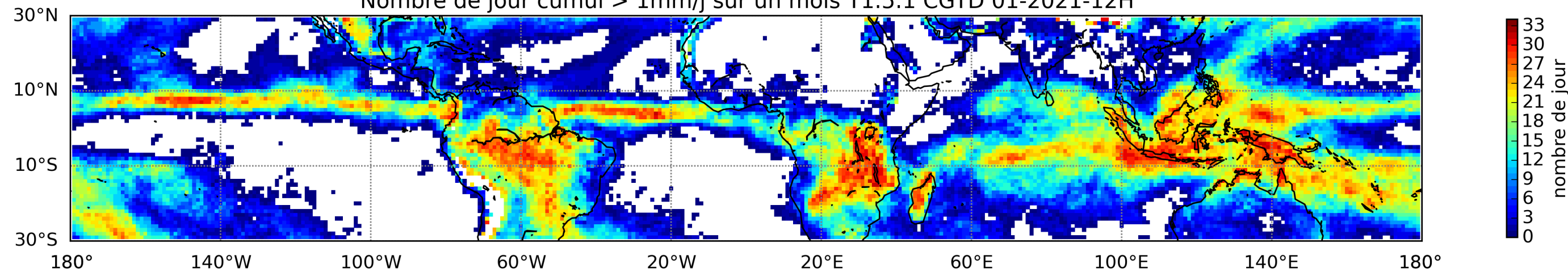
Nombre de jour cumul > 1mm/j sur un mois T1.5.1 CGTD 01-2021-12H
