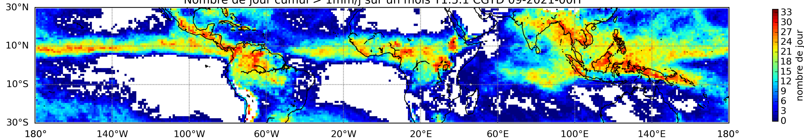
Nombre de jour cumul > 1mm/j sur un mois T1.5.1 CGTD 09-2021-00H
