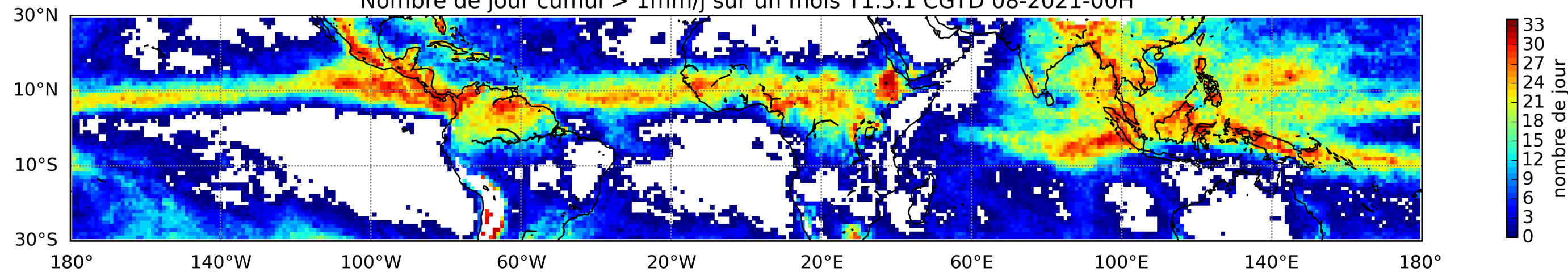
Nombre de jour cumul > 1mm/j sur un mois T1.5.1 CGTD 08-2021-00H
