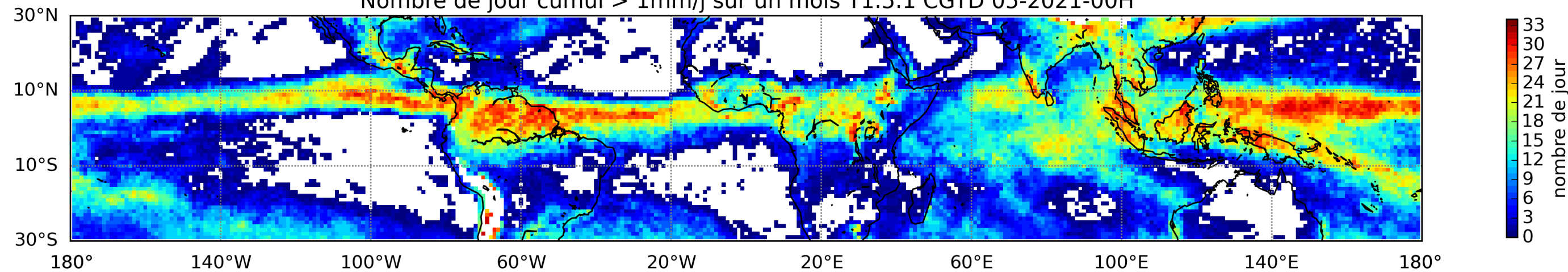
Nombre de jour cumul > 1mm/j sur un mois T1.5.1 CGTD 05-2021-00H
