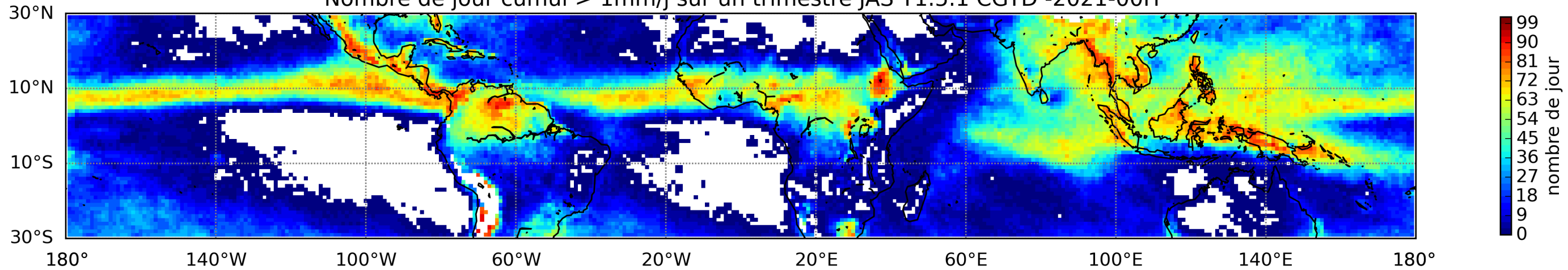
Nombre de jour cumul > 1mm/j sur un trimestre JAS T1.5.1 CGTD -2021-00H
