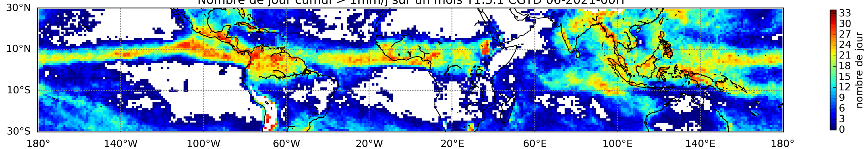
Nombre de jour cumul > 1mm/j sur un mois T1.5.1 CGTD 06-2021-00H
