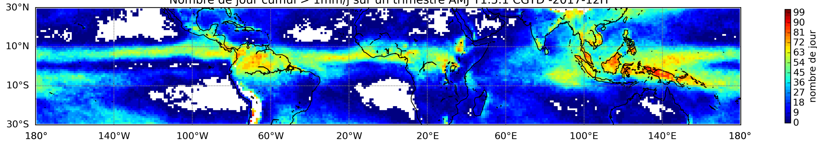
Nombre de jour cumul > 1mm/j sur un trimestre AMJ T1.5.1 CGTD -2017-12H
