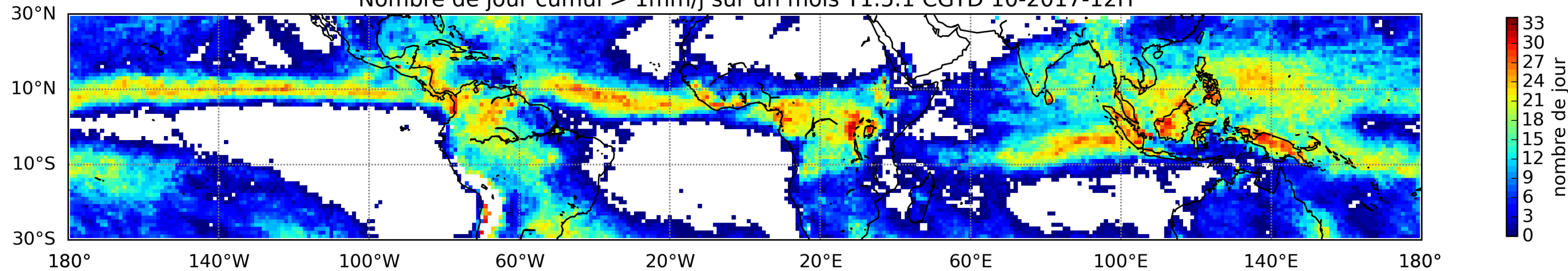
Nombre de jour cumul > 1mm/j sur un mois T1.5.1 CGTD 10-2017-12H
