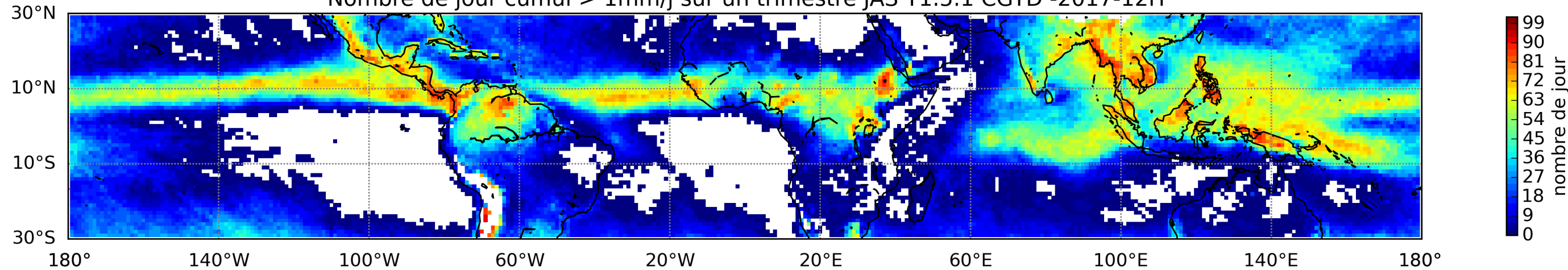
Nombre de jour cumul > 1mm/j sur un trimestre JAS T1.5.1 CGTD -2017-12H
