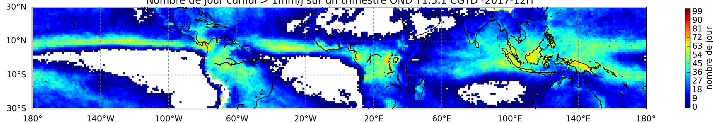
Nombre de jour cumul > 1mm/j sur un trimestre OND T1.5.1 CGTD -2017-12H
