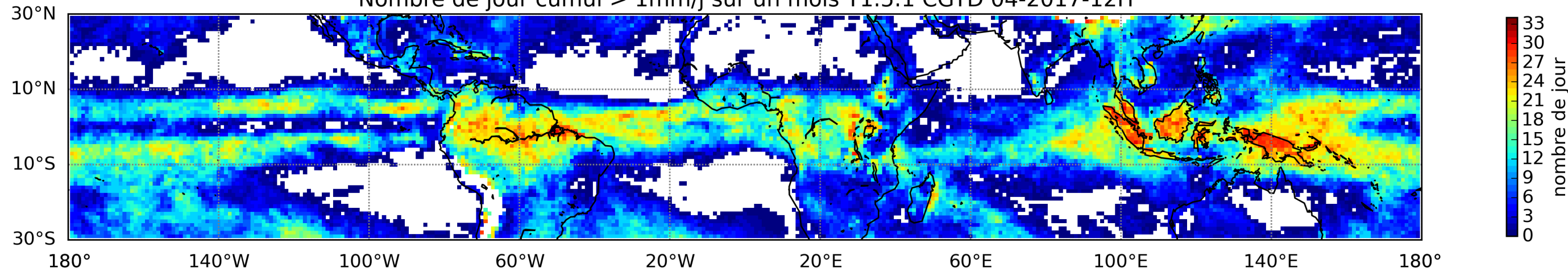
Nombre de jour cumul > 1mm/j sur un mois T1.5.1 CGTD 04-2017-12H
