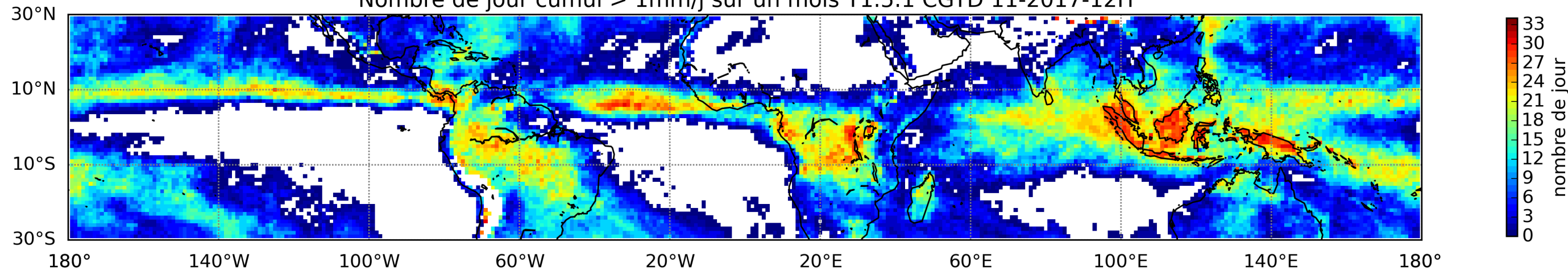
Nombre de jour cumul > 1mm/j sur un mois T1.5.1 CGTD 11-2017-12H
