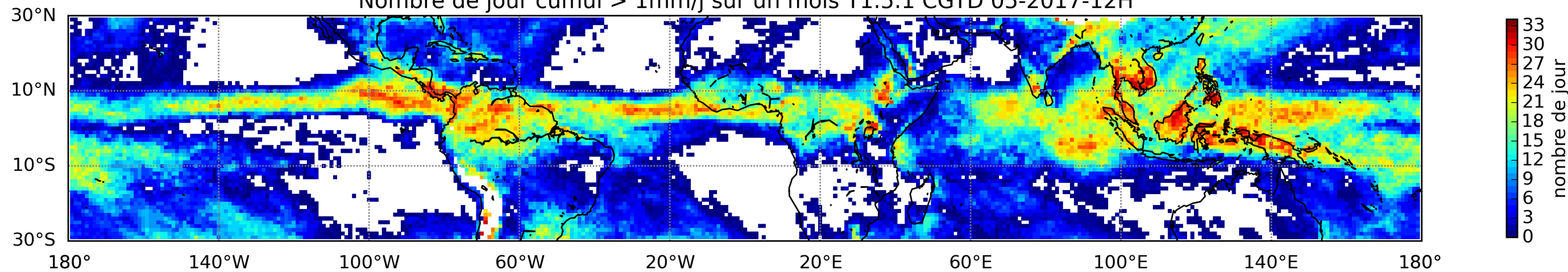
Nombre de jour cumul > 1mm/j sur un mois T1.5.1 CGTD 05-2017-12H
