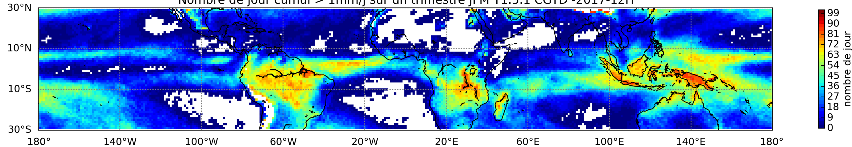
Nombre de jour cumul > 1mm/j sur un trimestre JFM T1.5.1 CGTD -2017-12H
