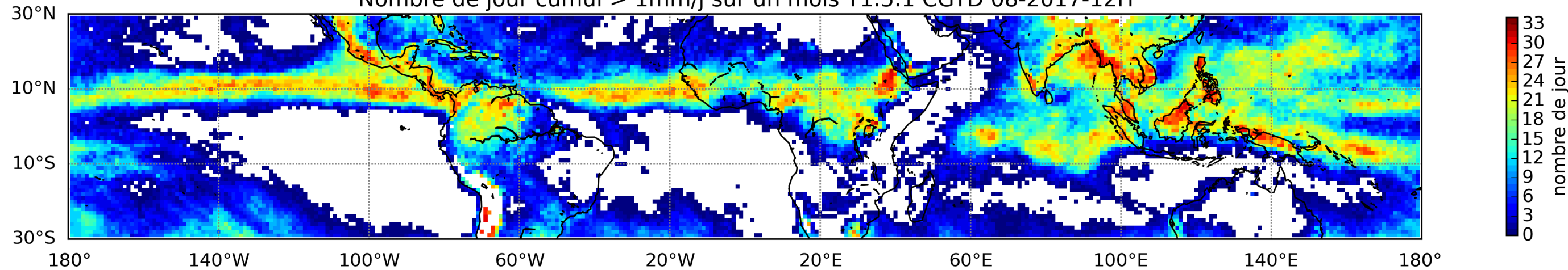
Nombre de jour cumul > 1mm/j sur un mois T1.5.1 CGTD 08-2017-12H
