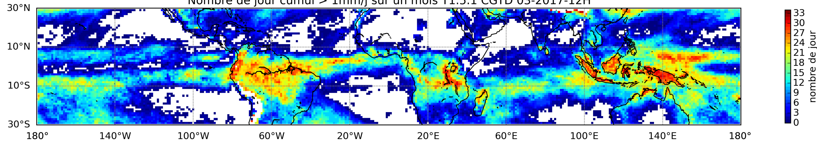
Nombre de jour cumul > 1mm/j sur un mois T1.5.1 CGTD 03-2017-12H
