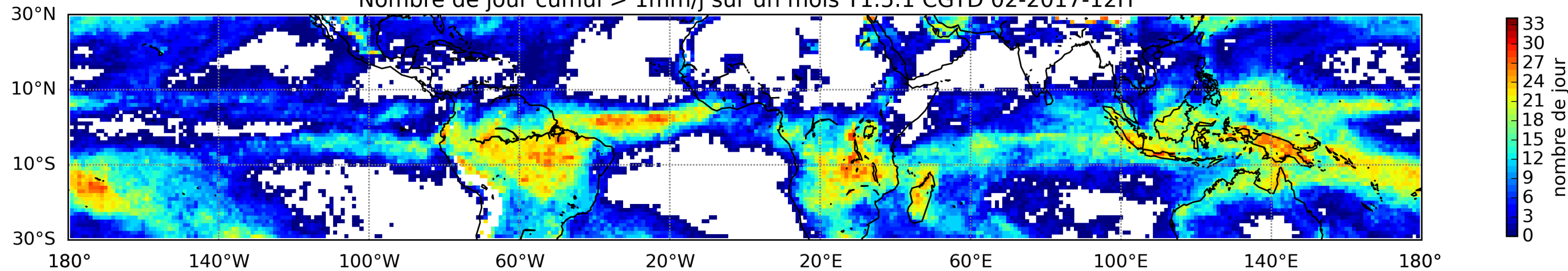
Nombre de jour cumul > 1mm/j sur un mois T1.5.1 CGTD 02-2017-12H
