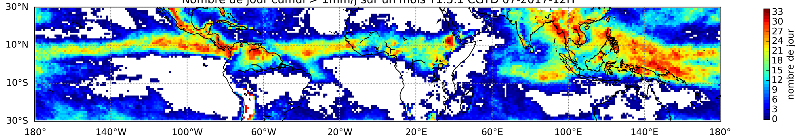
Nombre de jour cumul > 1mm/j sur un mois T1.5.1 CGTD 07-2017-12H
