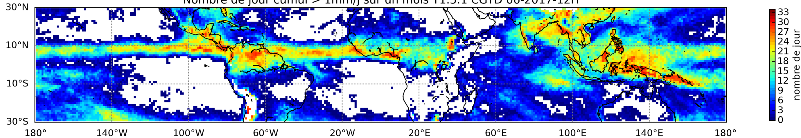
Nombre de jour cumul > 1mm/j sur un mois T1.5.1 CGTD 06-2017-12H
