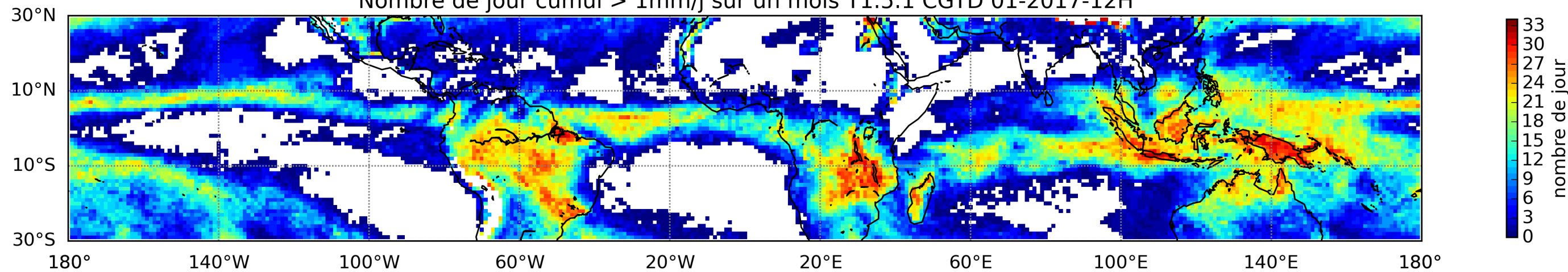
Nombre de jour cumul > 1mm/j sur un mois T1.5.1 CGTD 01-2017-12H
