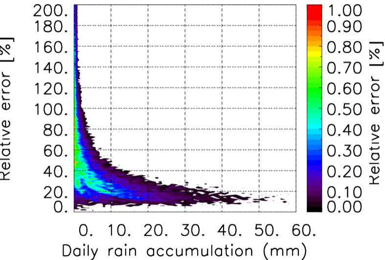
TERRE : 12 2017 12H
