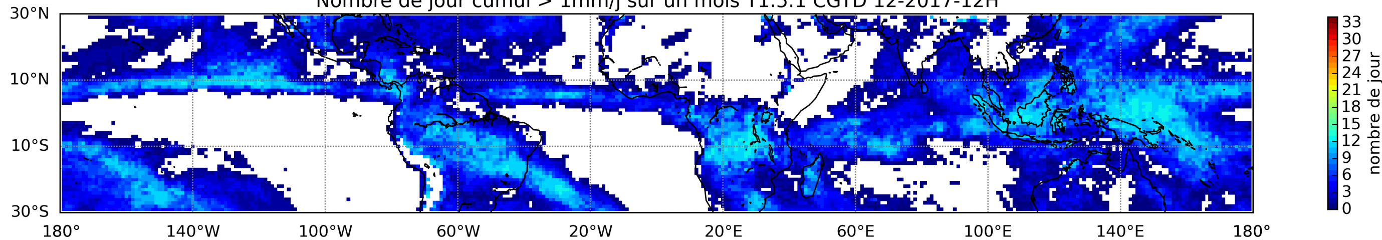
Nombre de jour cumul > 1mm/j sur un mois T1.5.1 CGTD 12-2017-12H
