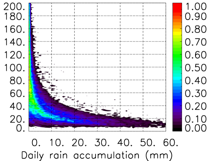
MER : 12 2017 12H
