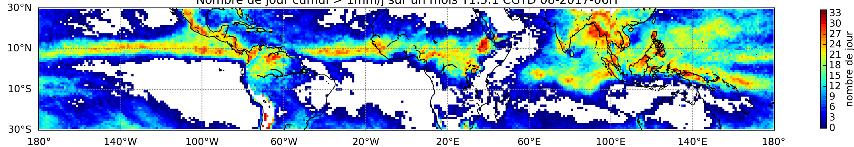
Nombre de jour cumul > 1mm/j sur un mois T1.5.1 CGTD 08-2017-06H
