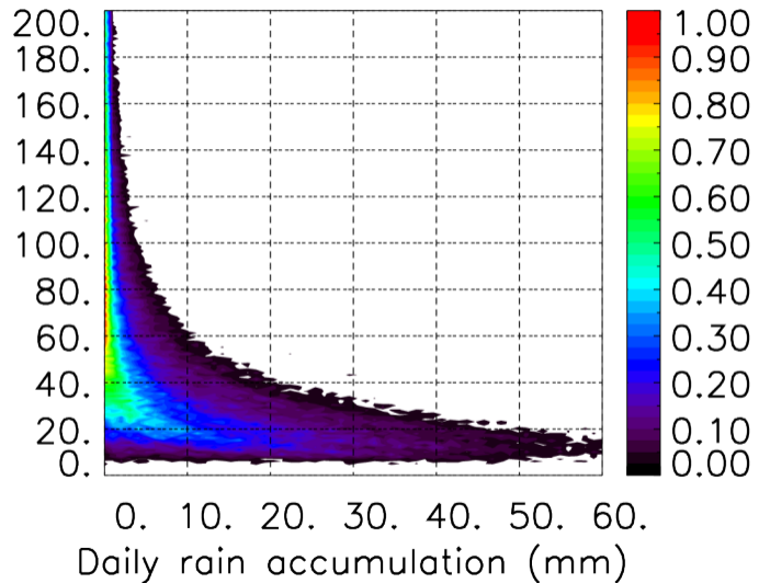
MER : 09 2017 06H
