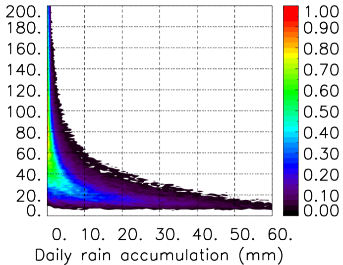
MER : 10 2017 06H
