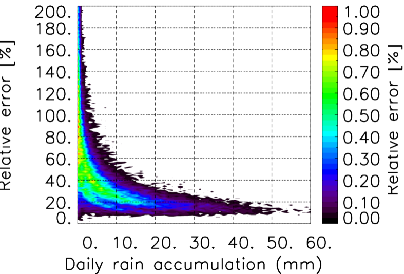
TERRE : 07 2017 06H
