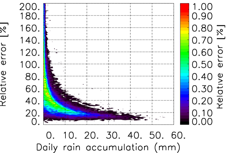
TERRE : 10 2017 06H
