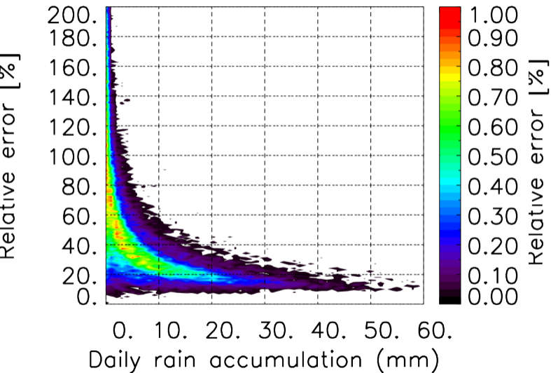
TERRE : 06 2017 06H
