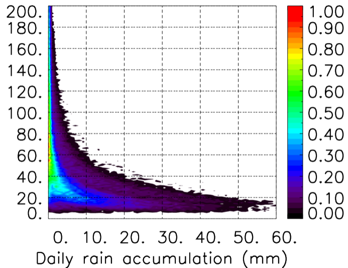
MER : 07 2017 06H
