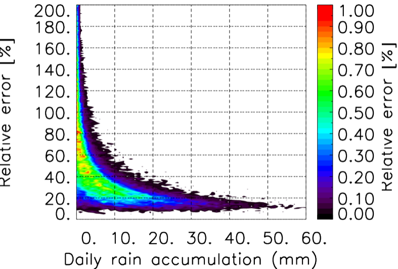
TERRE : 09 2017 06H
