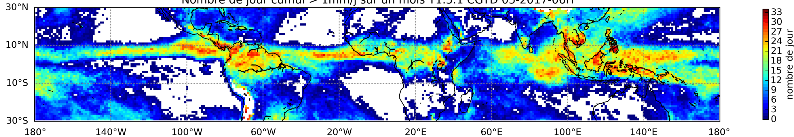
Nombre de jour cumul > 1mm/j sur un mois T1.5.1 CGTD 05-2017-06H
