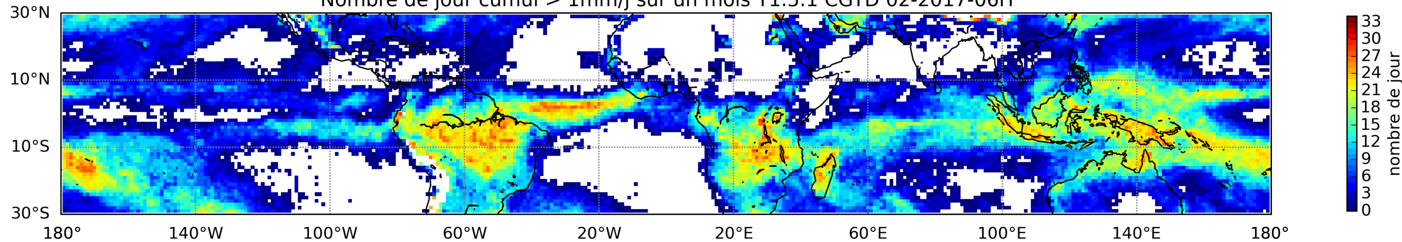
Nombre de jour cumul > 1mm/j sur un mois T1.5.1 CGTD 02-2017-06H
