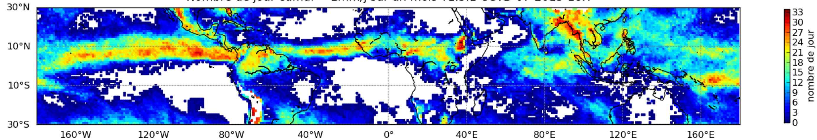
Nombre de jour cumul > 1mm/j sur un mois T1.5.1 CGTD 07-2015-18H
