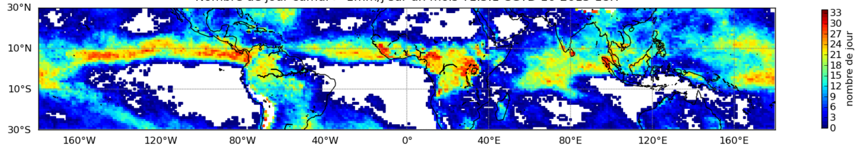
Nombre de jour cumul > 1mm/j sur un mois T1.5.1 CGTD 10-2015-18H
