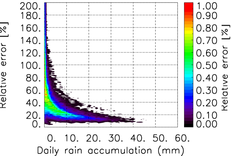
TERRE : 12 2015 00H
