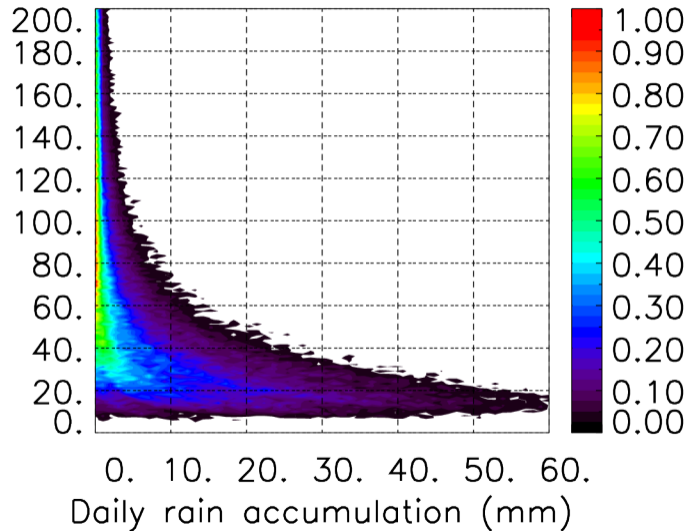
MER : 08 2012 06H
