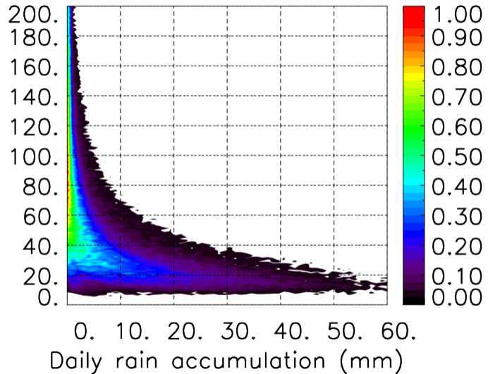
MER : 07 2012 06H
