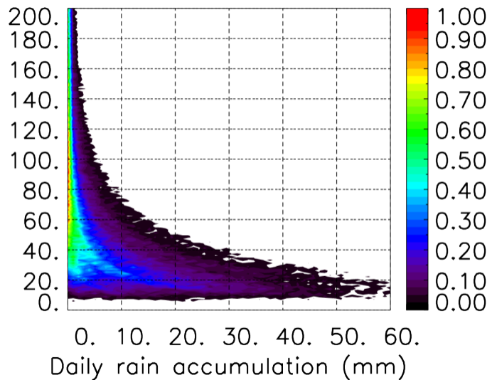
MER : 11 2012 06H
