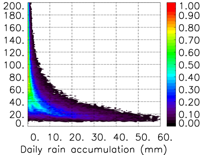
MER : 09 2012 06H
