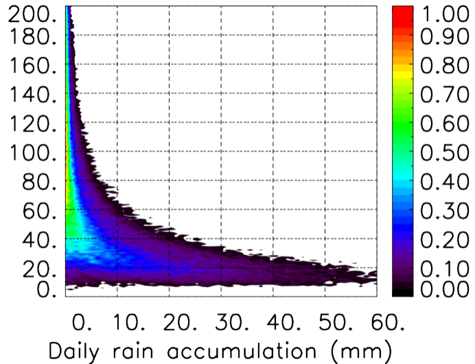
MER : 10 2012 06H
