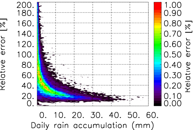
TERRE : 09 2012 06H
