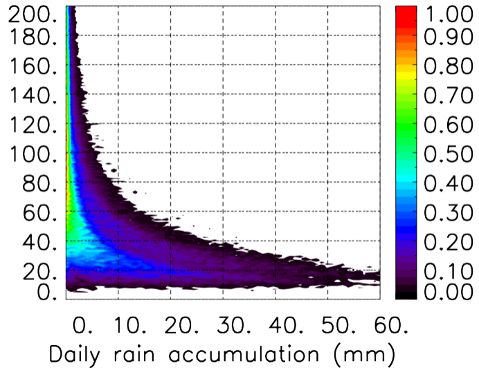
MER : 12 2012 06H
