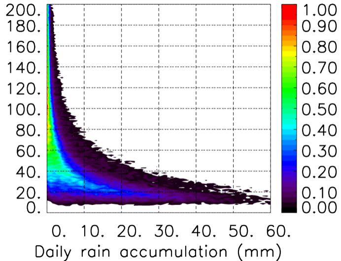
MER : 05 2012 06H
