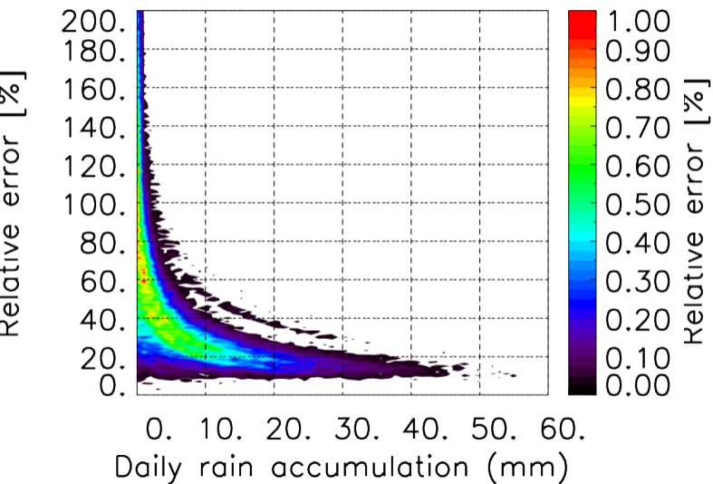
TERRE : 11 2012 06H
