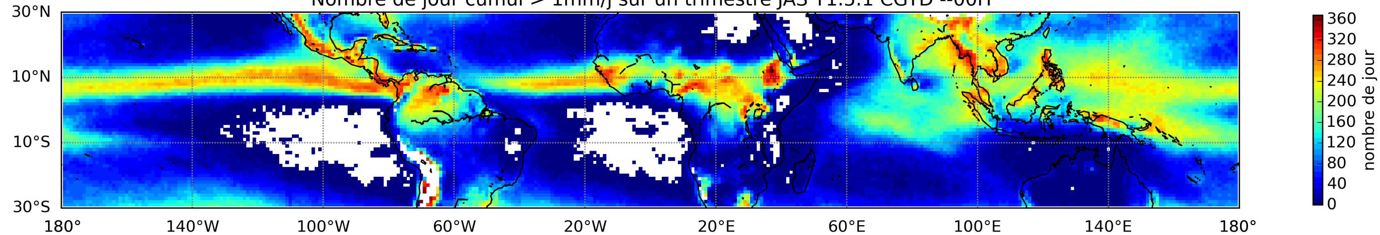
Nombre de jour cumul > 1mm/j sur un trimestre JAS T1.5.1 CGTD --00H
