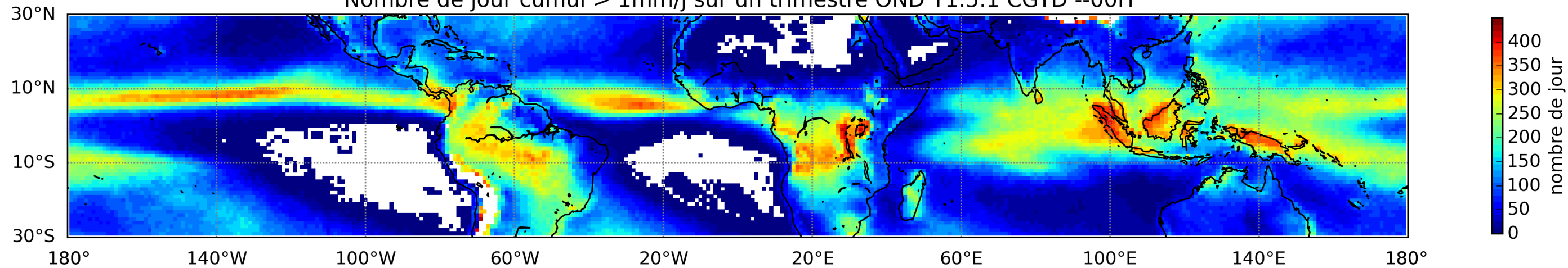
Nombre de jour cumul > 1mm/j sur un trimestre OND T1.5.1 CGTD --00H
