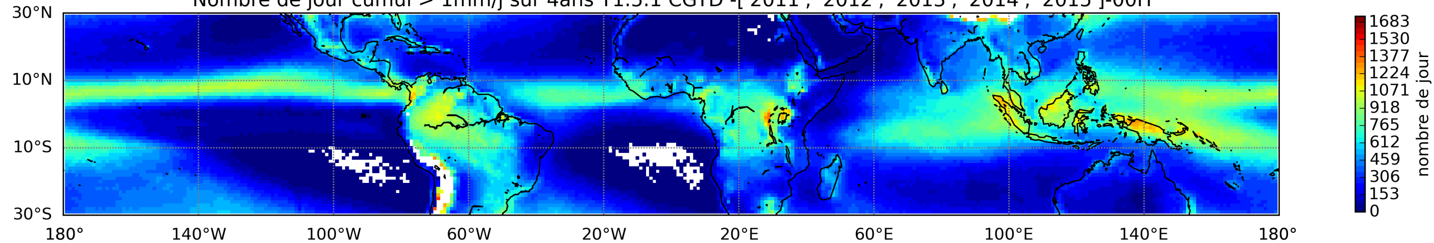
Nombre de jour cumul > 1mm/j sur 4ans T1.5.1 CGTD -['2011', '2012', '2013', '2014', '2015']-00H
