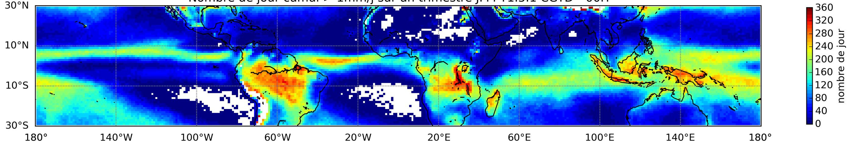
Nombre de jour cumul > 1mm/j sur un trimestre JFM T1.5.1 CGTD --00H
