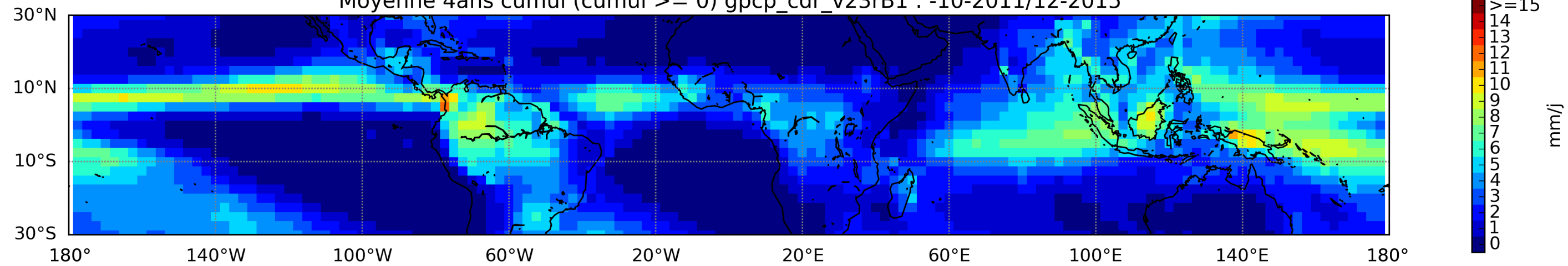
Moyenne 4ans cumul (cumul \geq 0 ) gpcp_cdr_v23rB1 : -10-2011/12-2015
