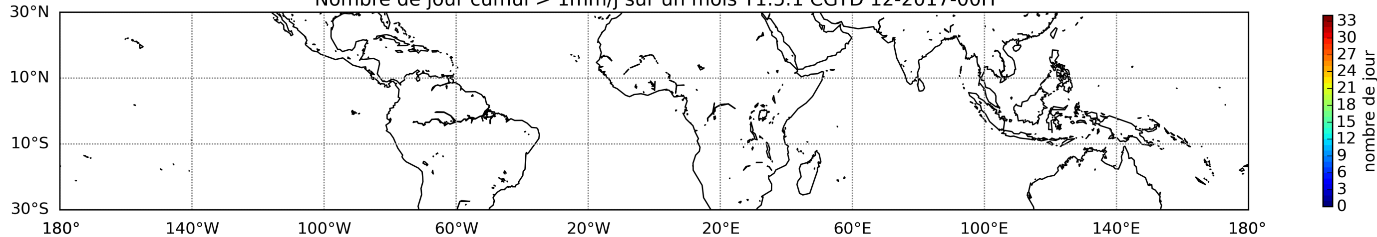
Nombre de jour cumul > 1mm/j sur un mois T1.5.1 CGTD 12-2017-00H
